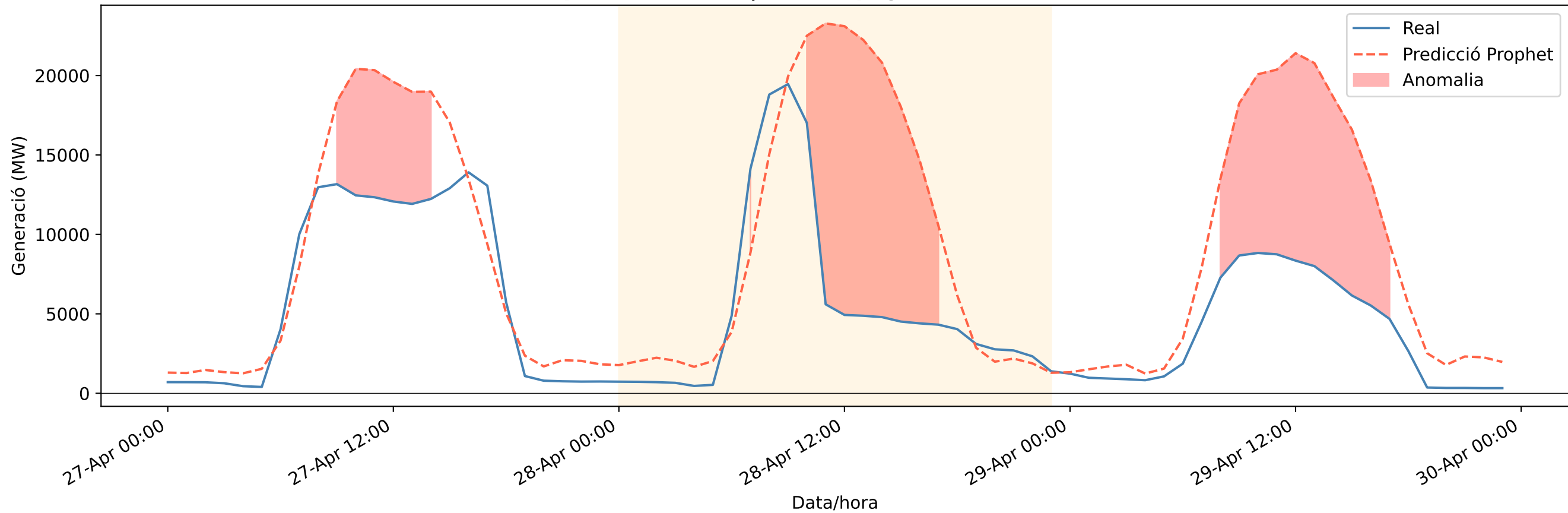
Prophet - Solar PV | Detall apagada 27-29 abril 2025
