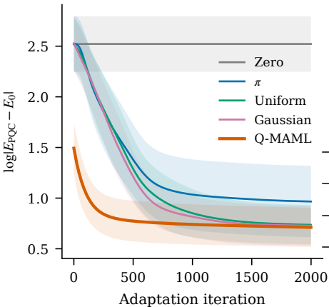
a Heisenberg XYZ, 6 qubits
