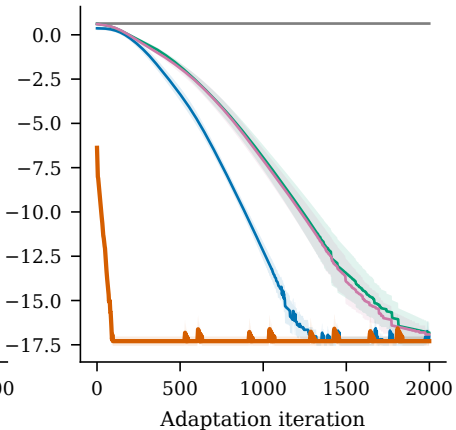
b \text{H}_2 molecule, 4 qubits
