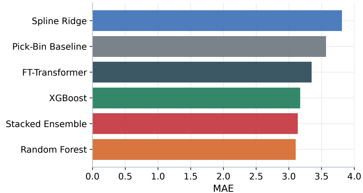
MAE
