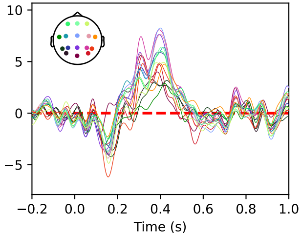
overt VSA
