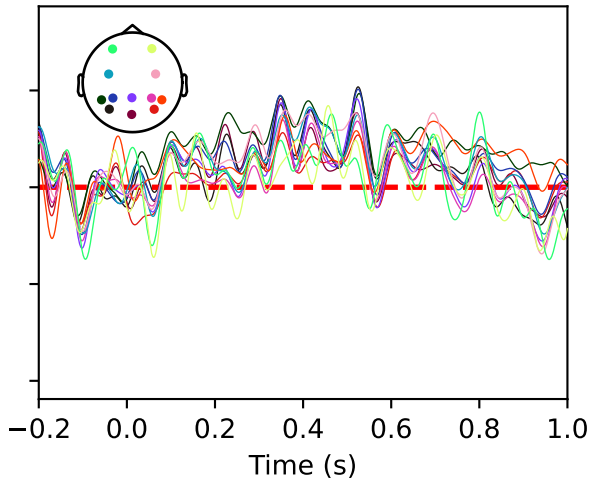
covert VSA
