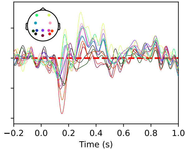
free VSA
