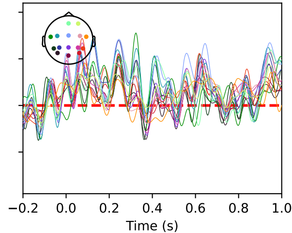
free VSA
