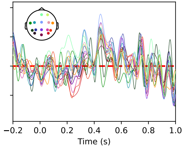
covert VSA
