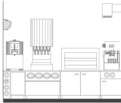
1 Elevation 1 1:50
