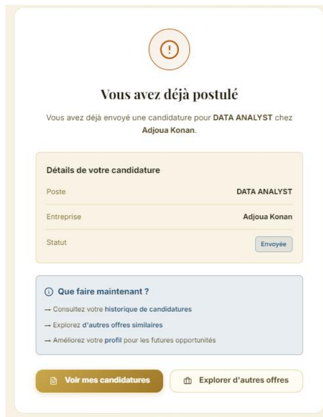
Figure 25 : Candidature envoyée
