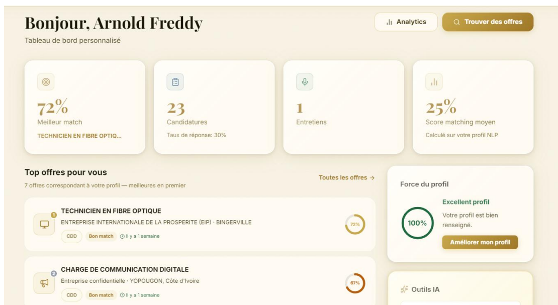
Figure 23 : Dashboard utilisateur
