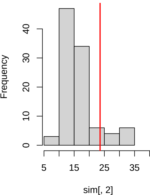
SE of Simple estimates
