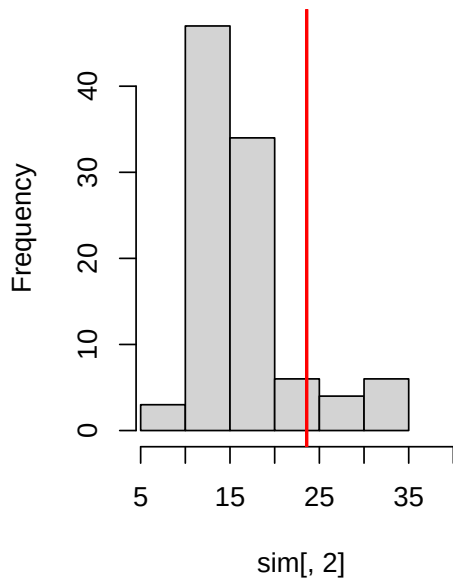
SE of Simple estimates
