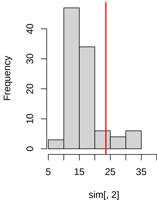
SE of Simple estimates
