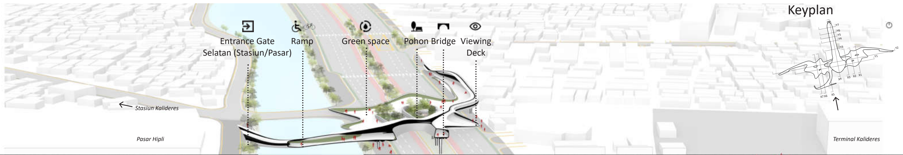
Potongan Perspektif (X5)
