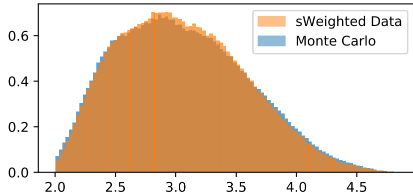
mu_ETA
