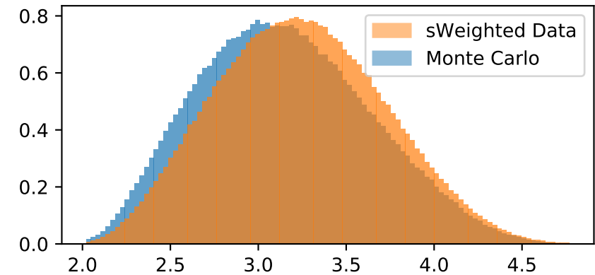
D0_ETA
