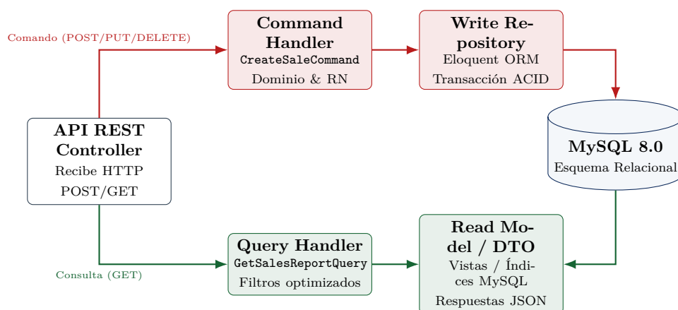
Figura 3: Flujo de Ejecución de Comandos y Consultas (CQRS) en SYSELL.
