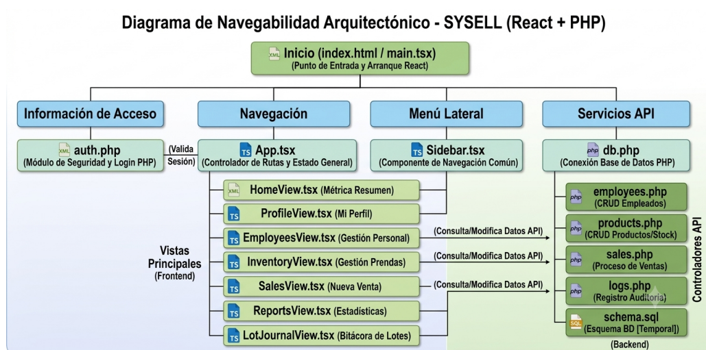
Figura 11: Diagrama de Navegabilidad y Flujo de Vistas del Sistema SYSELL.
