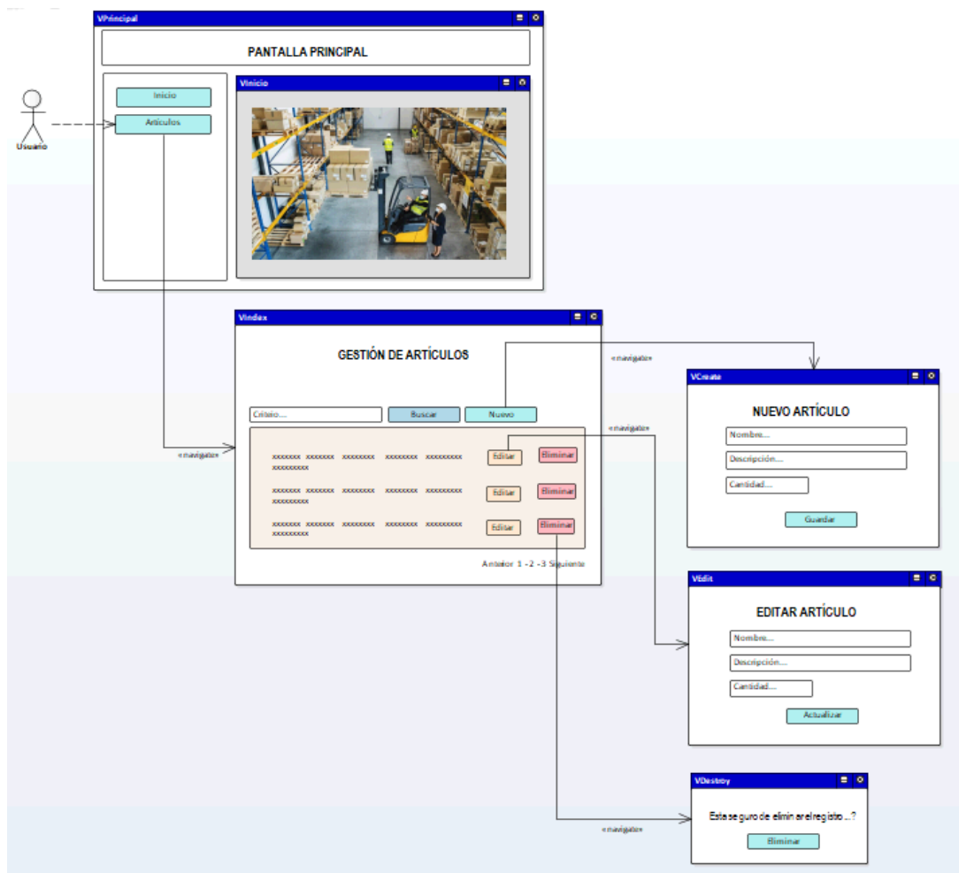
PROTOTIPO: Gestionar Artículos de Almacén
