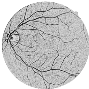
Frangi p
