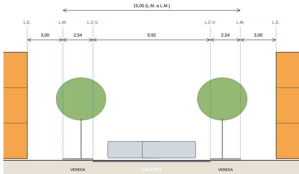
PERFIL VIAL TIPO · CALLE LOCAL · ESC. 1/200
