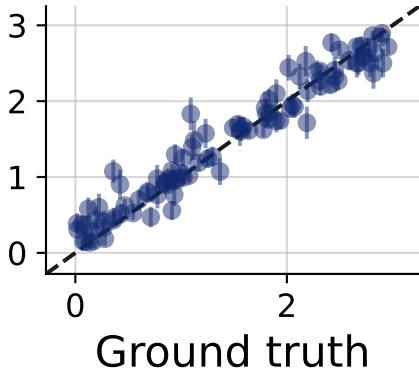
NPE
