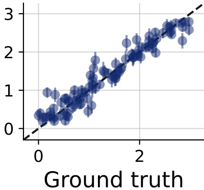
NPE
