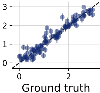
STAN
