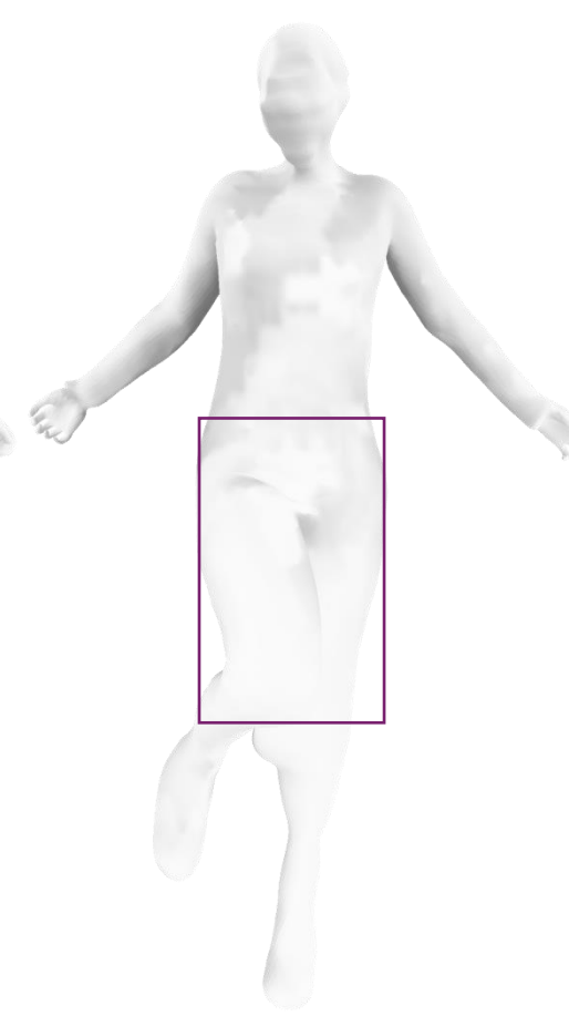
GS-IR + template
