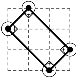
Rectangle Té els quatre angles iguals.
