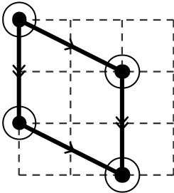
Paral·lelogram Té dos parells de costats paral·lels.
