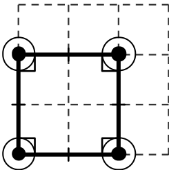
Quadrat Té els quatre costats iguals i els quatre angles iguals.
