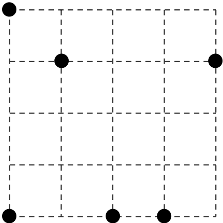
11 Triangle rectangle isòsceles
