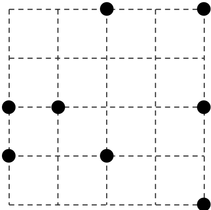
29 Triangle rectangle isòsceles
