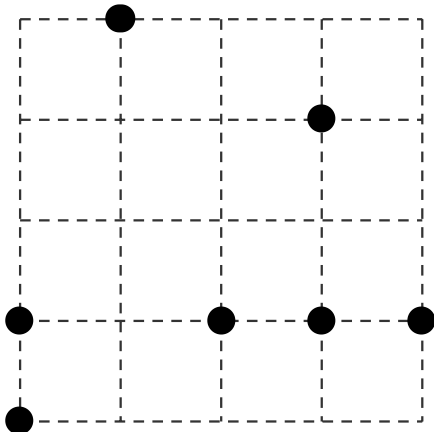
36 Triangle rectangle isòsceles
