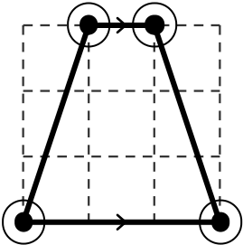
Trapezi Té un parell de costats paral·lels.
