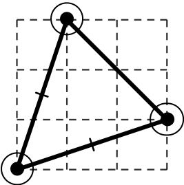
Triangle isòsceles Té dos costats iguals.
