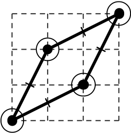
Rombe Té els quatre costats iguals.
