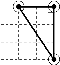
Triangle rectangle Té un angle recte.
