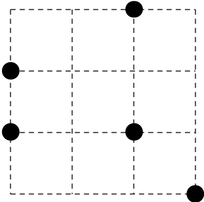
21 Triangle rectangle isòsceles
