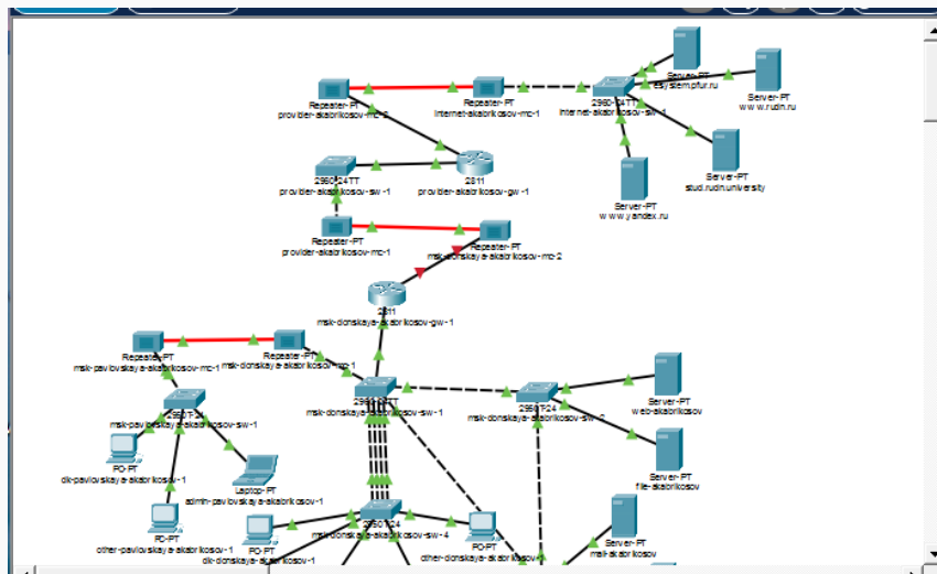
Рис. 1: Общая топология сети организации и провайдера
