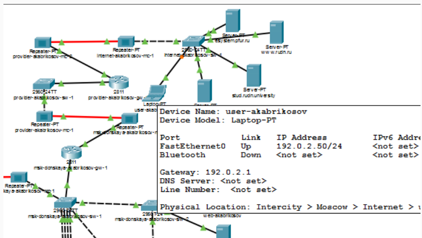
Рис. 14: Параметры внешнего клиента
