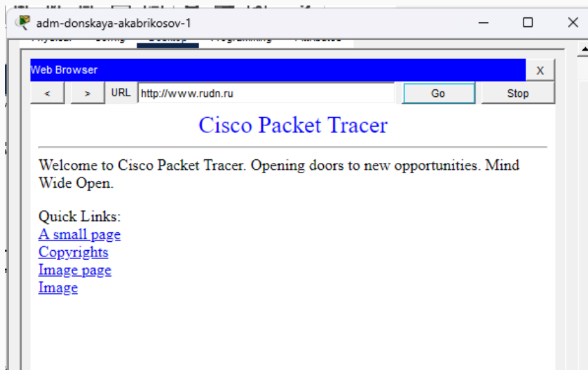
Рис. 11: Доступ к www.rudn.ru из сети администрации
