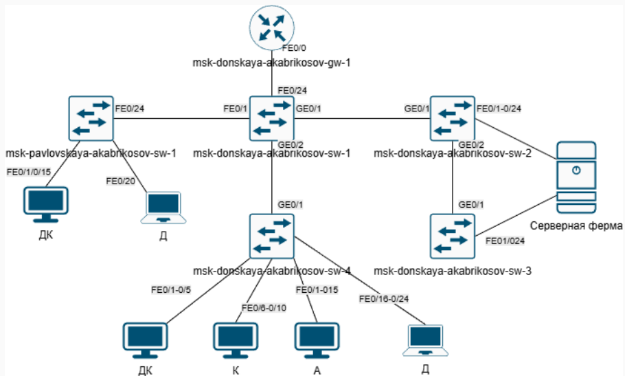
Рис. 1: Схема L1 — физическая топология
