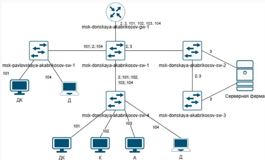
Рис. 2: Схема L2 — распределение VLAN
