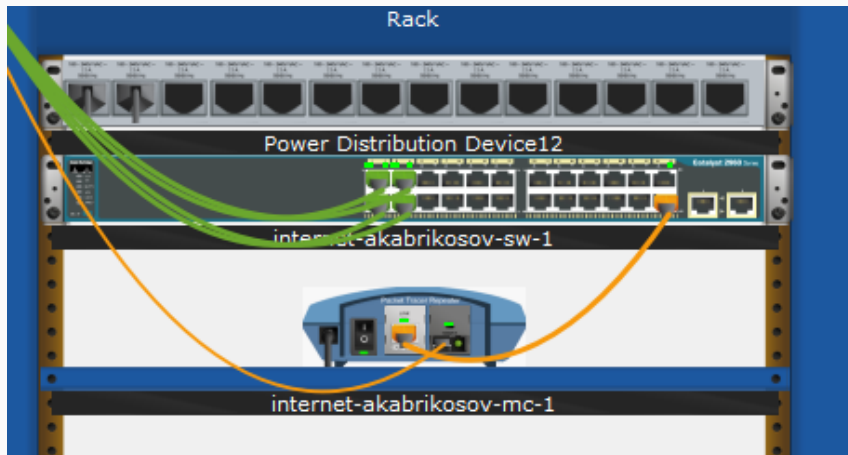
Рис. 8: Коммутатор Интернет-сети
