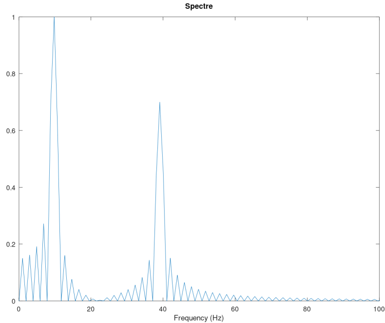
Рис. 2.8: Спектр суммы
