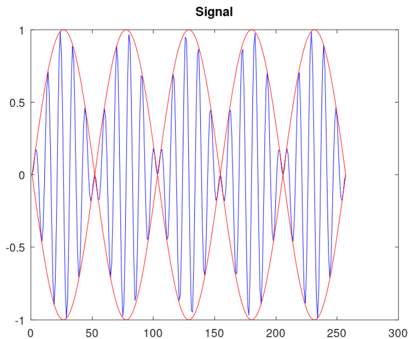
Рис. 2.9: АМ-сигнал и огибающая
