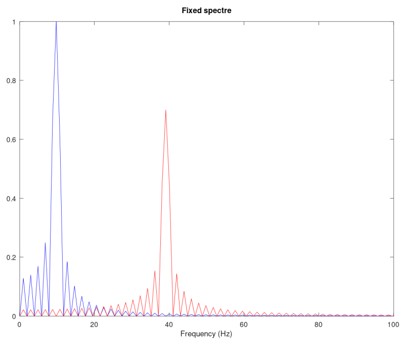
Рис. 2.6: Исправленный спектр
