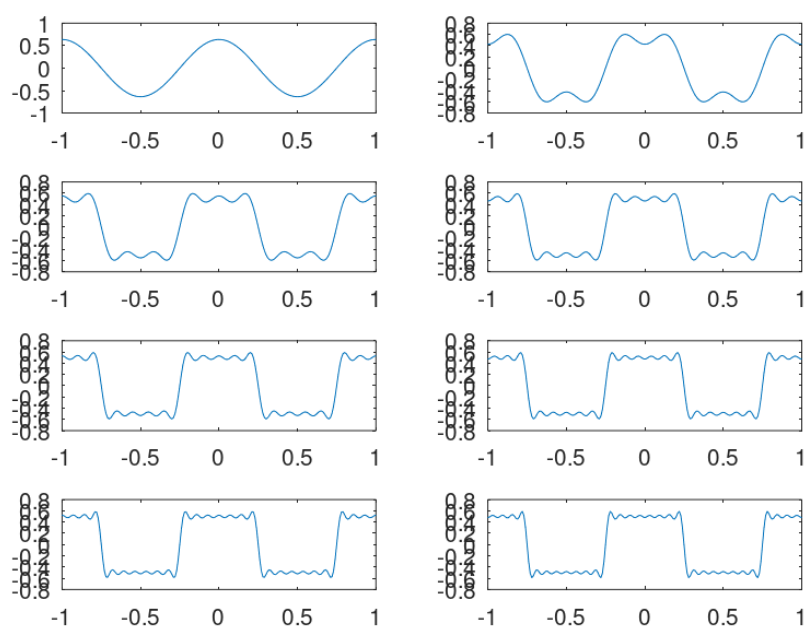
Рис. 2.3: Меандр через cos-ряд ( N=1\dots 8 )
