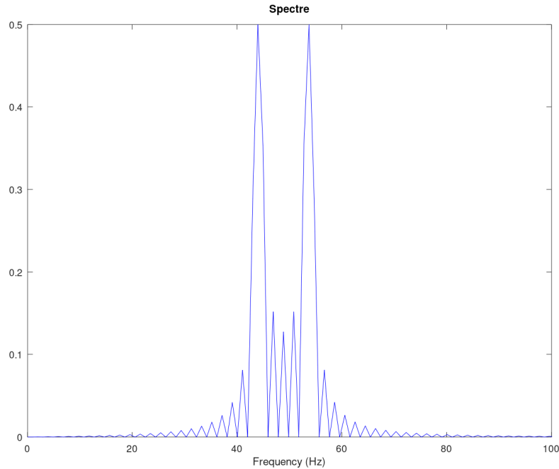
Рис. 2.10: Спектр АМ-сигнала
