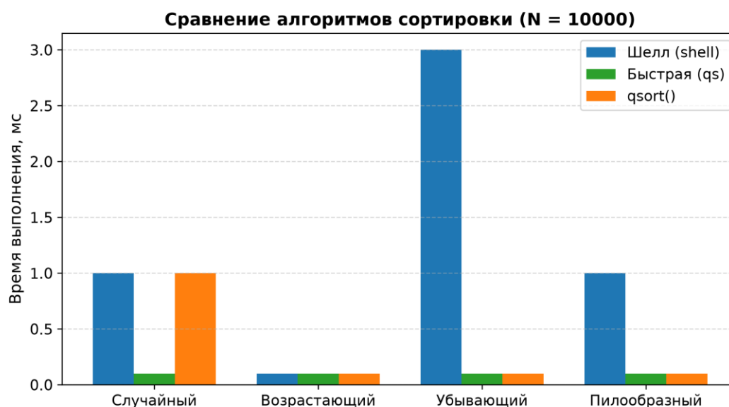
Рисунок 2 – Сравнение времени работы алгоритмов сортировки (N = 10000)
