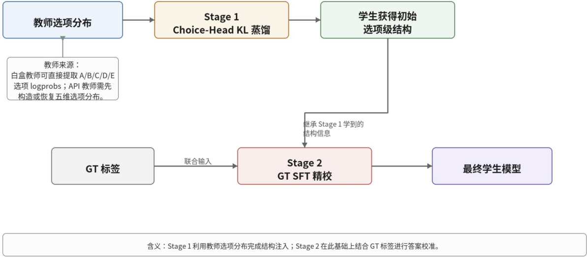
图 3-1 Choice-Head 两阶段蒸馏流程图。
