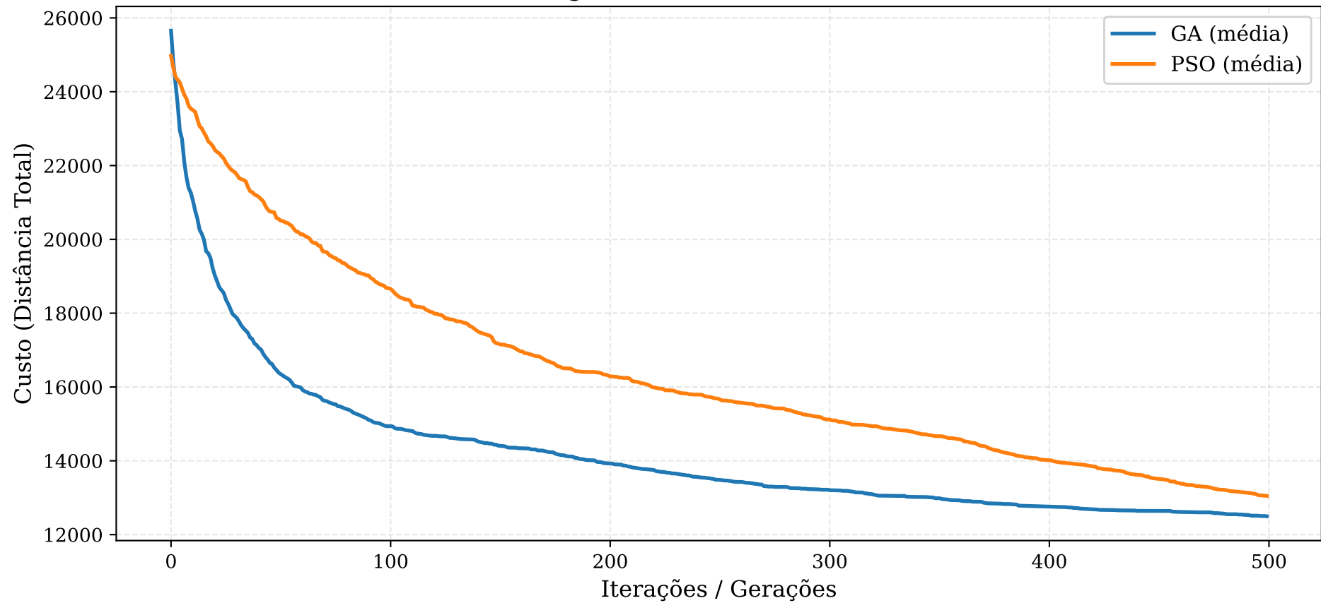
Convergência - berlin52 (52 cidades)
