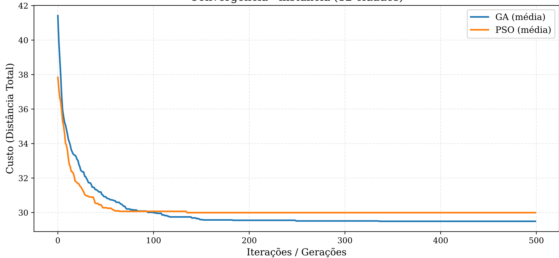
Convergência - instancia (12 cidades)
