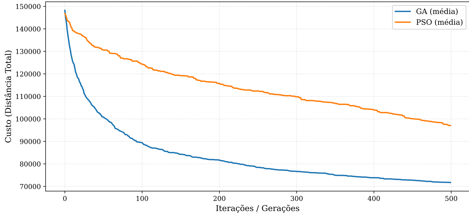
Convergência - kroA100 (100 cidades)
