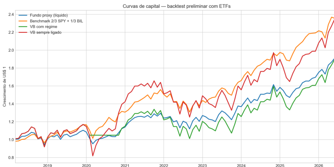
Figura 1. Curvas de capital do fundo proxy, benchmark e VB.
