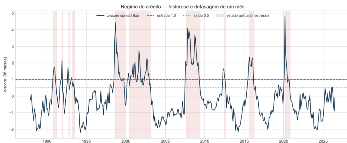
Figura 2. Z-score do BAA10Y, limiares de histerese e meses de estresse.
