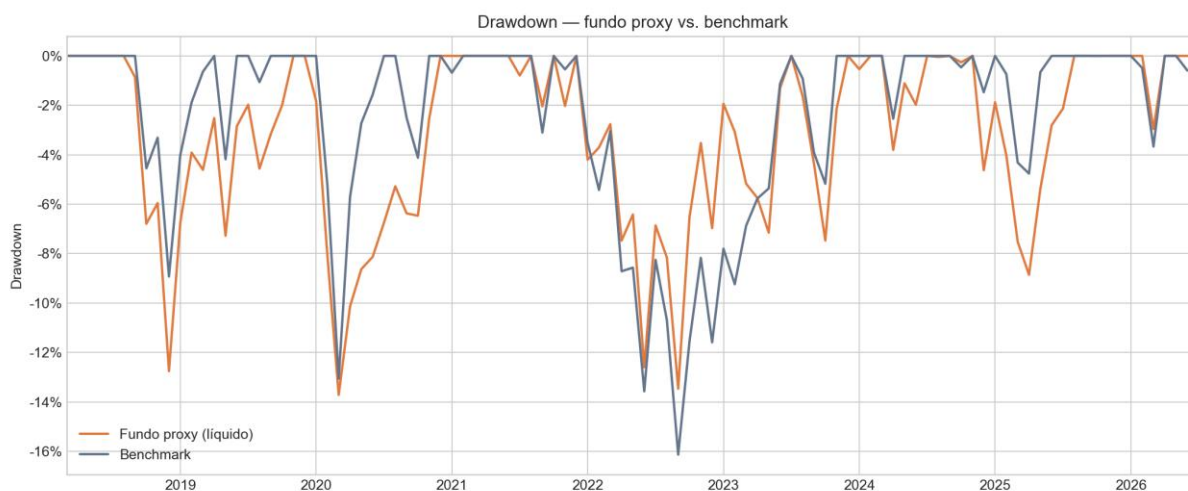
Figura 4. Drawdown do fundo proxy líquido e do benchmark.
