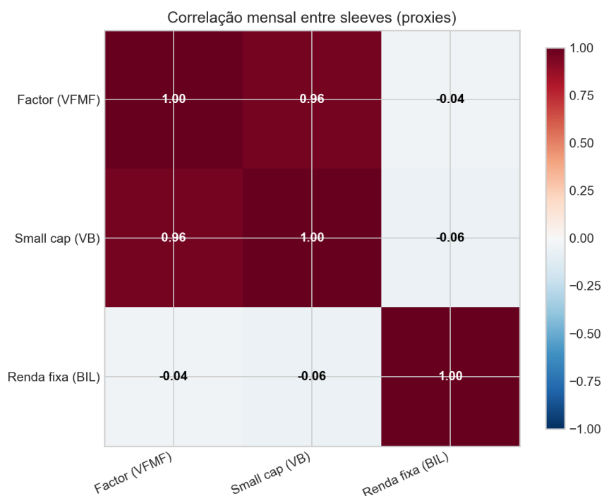
Figura 3. Correlação mensal entre os sleeves representados por ETFs.
