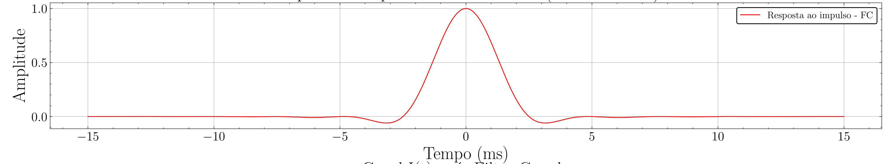
Resposta ao Impulso do Filtro Casado (RRC invertido)
