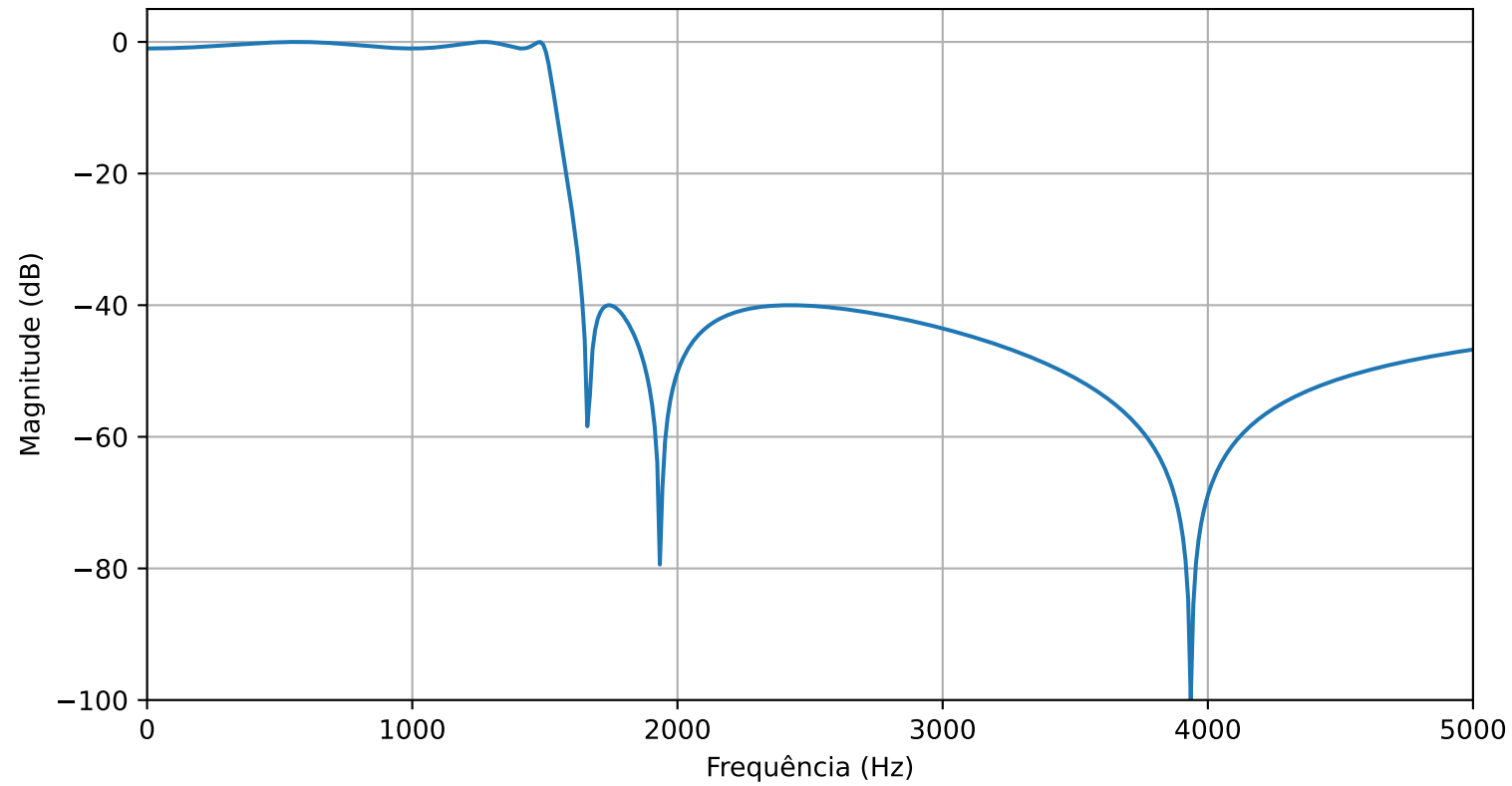
Elíptico
