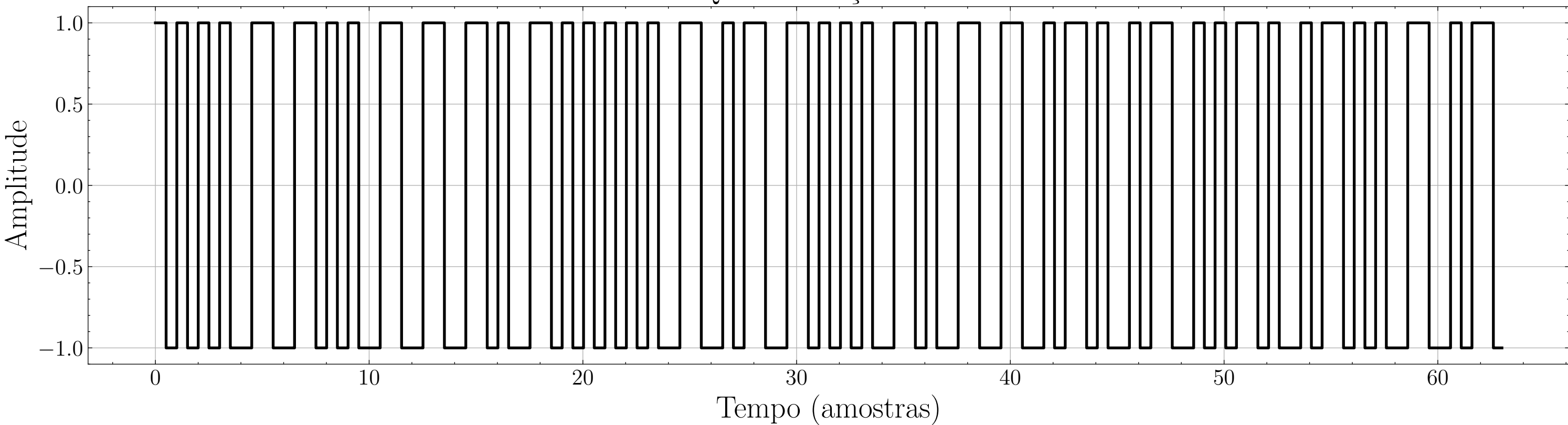
Canal Q - Codificação Manchester
