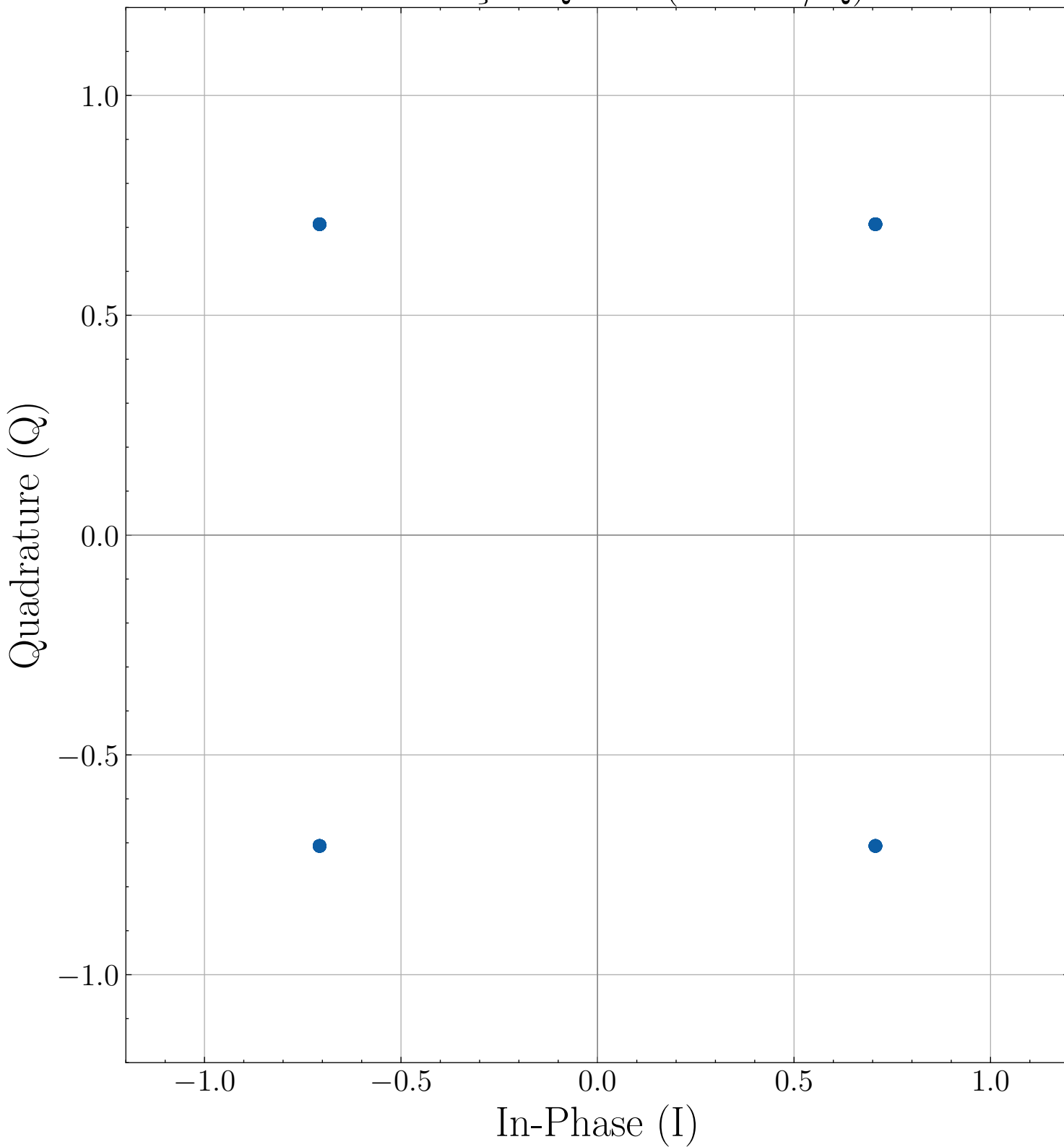
Constelação QPSK (Plano I/Q)
