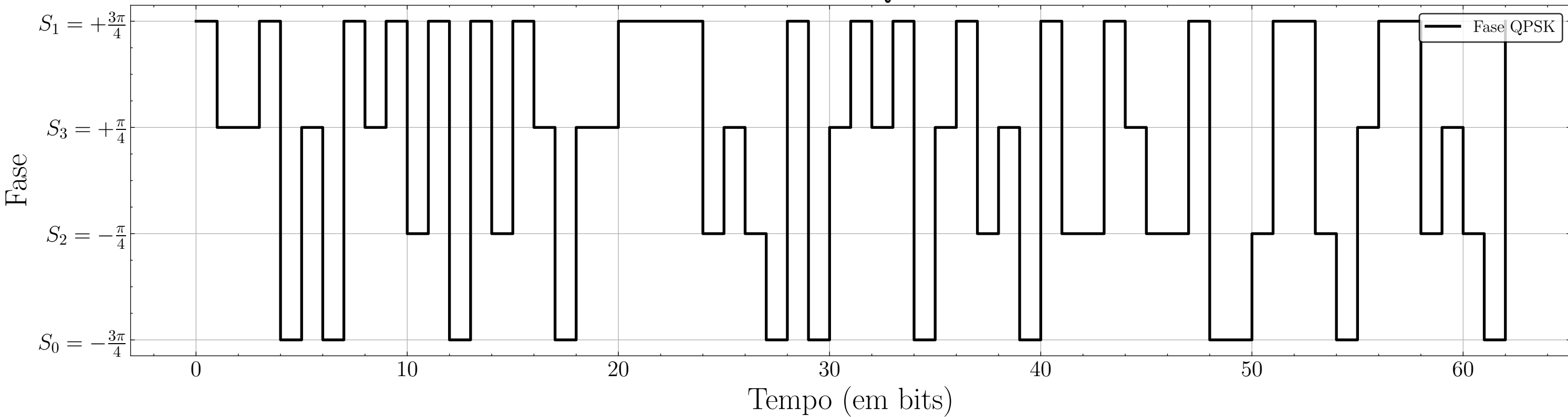
Símbolos QPSK
