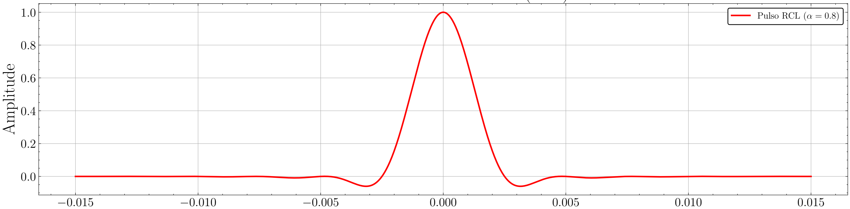
Pulso Raised Cosine Limitado (RCL)
