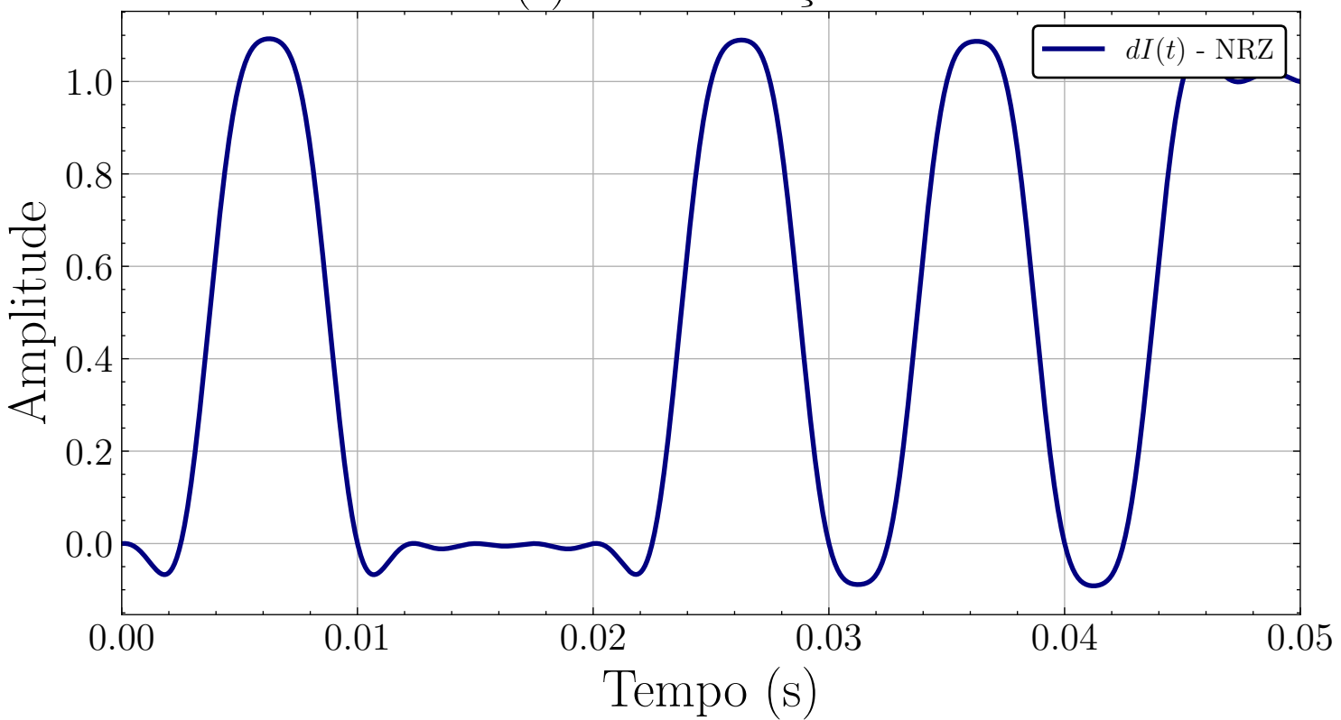
Sinal dI(t) - Formatação com RCL
