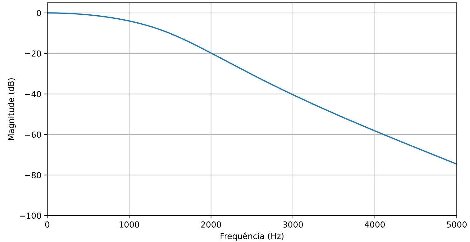
Bessel
