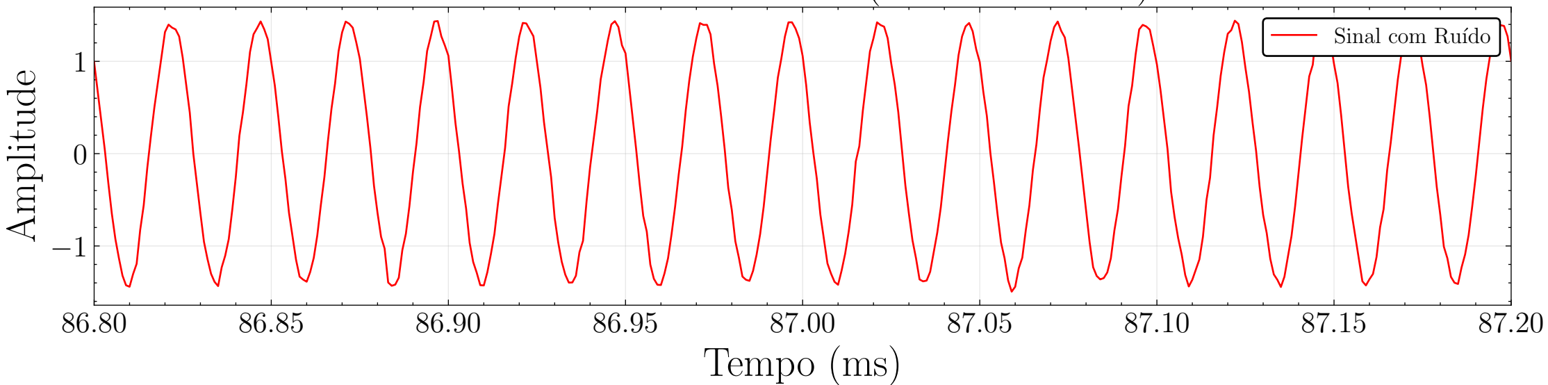
Sinal com Ruído AWGN (SNR = 25.0 dB)
