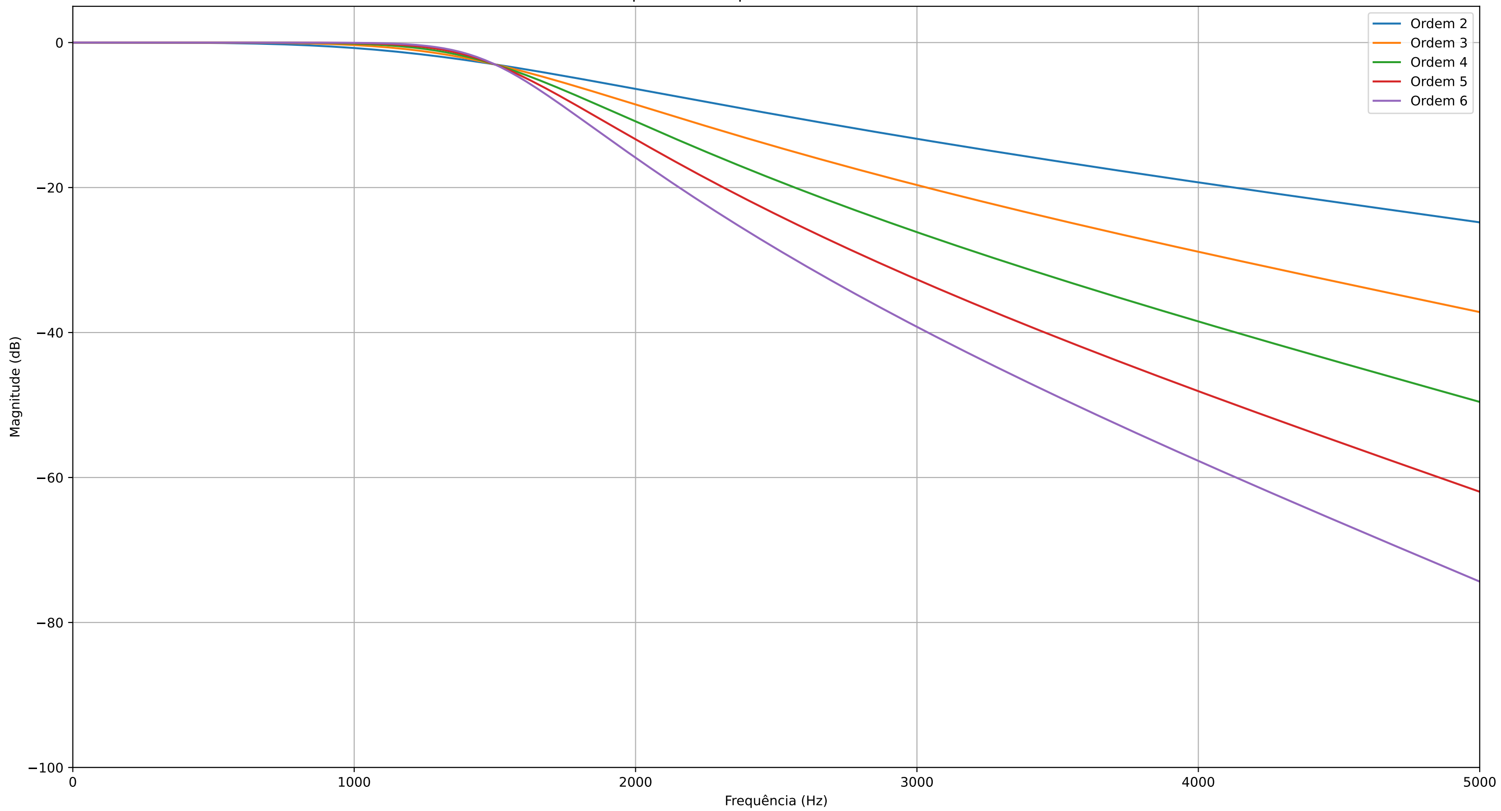
Resposta em frequência - Filtro Butterworth
