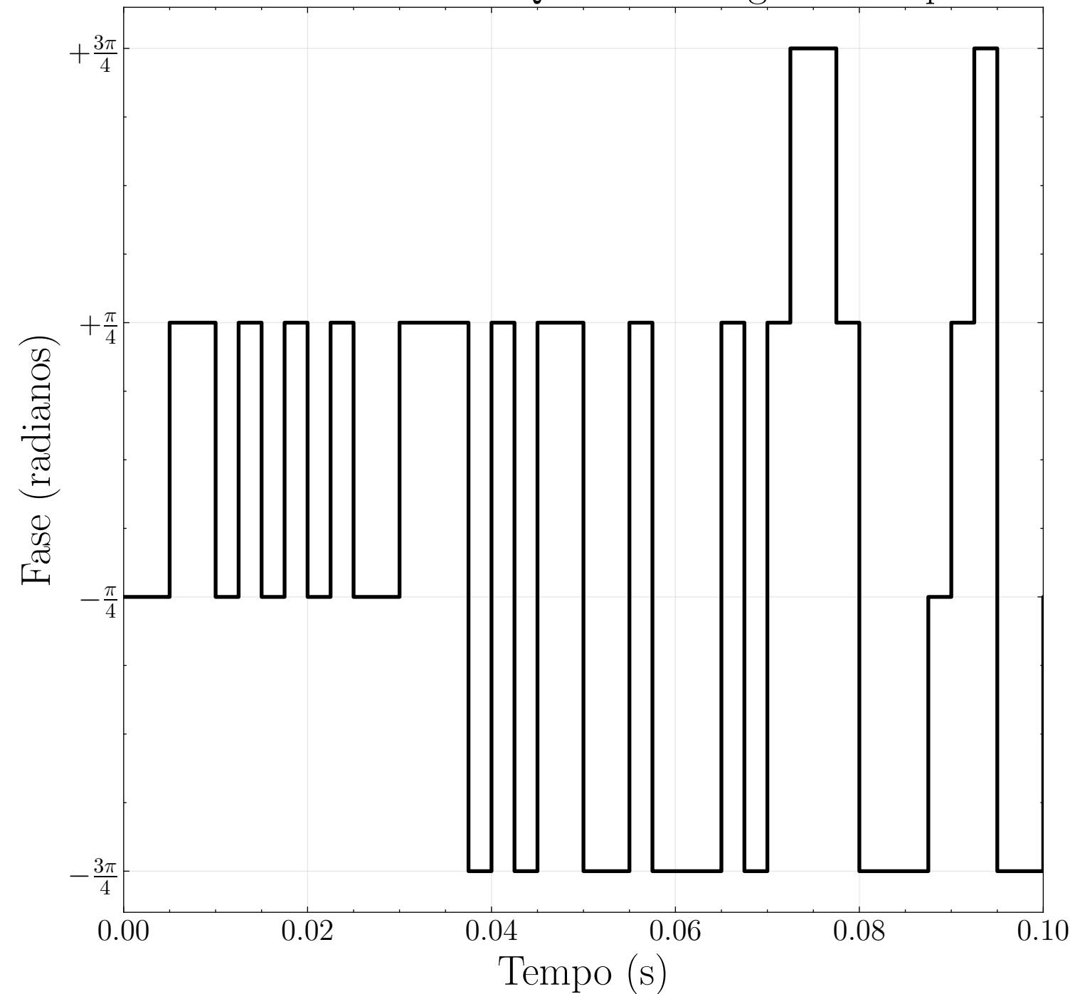
Fase dos Símbolos QPSK ao Longo do Tempo
