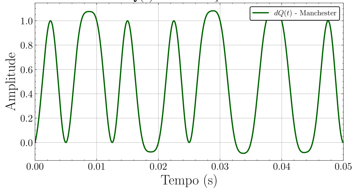
Sinal dQ(t) - Formatação com RCL
