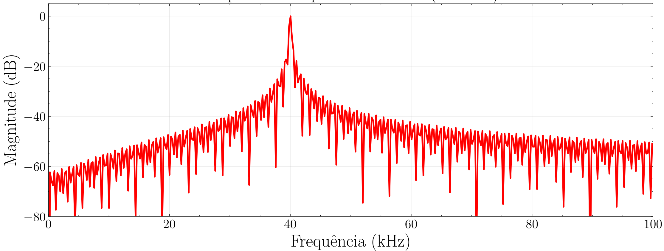
Resposta ao Impulso do Filtro Q (Seno)
