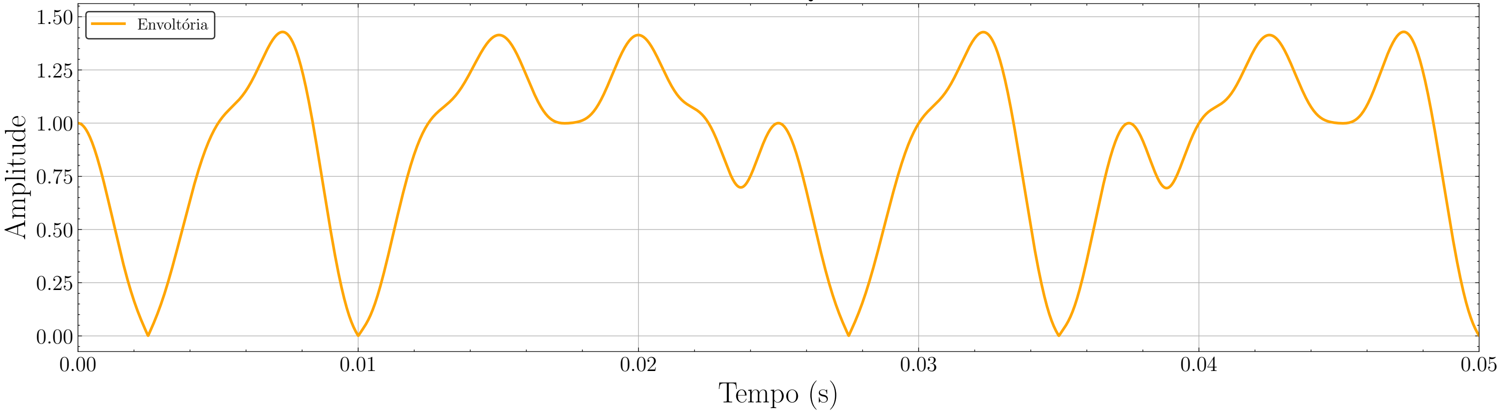
Envoltória do Sinal QPSK Modulado
