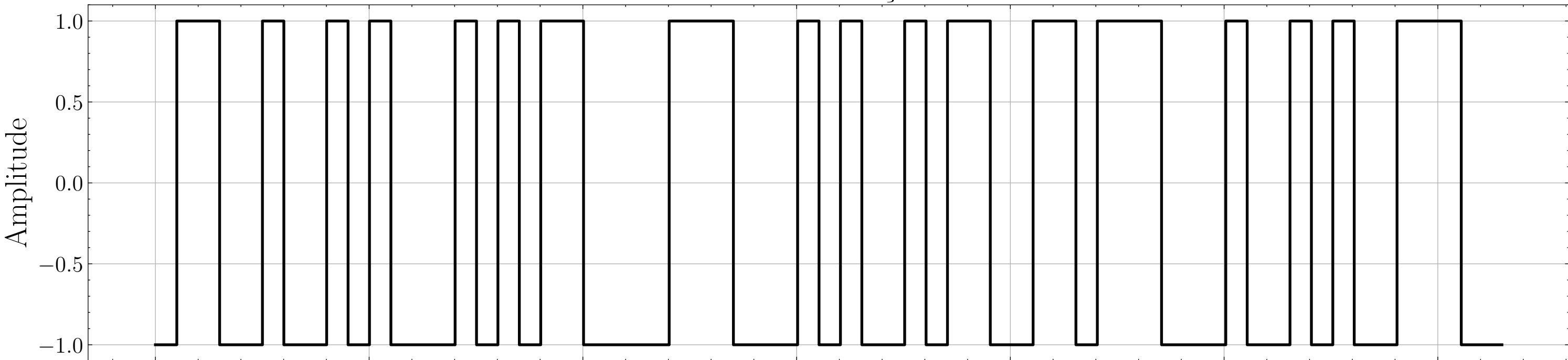
Canal Q - Codificação Manchester
