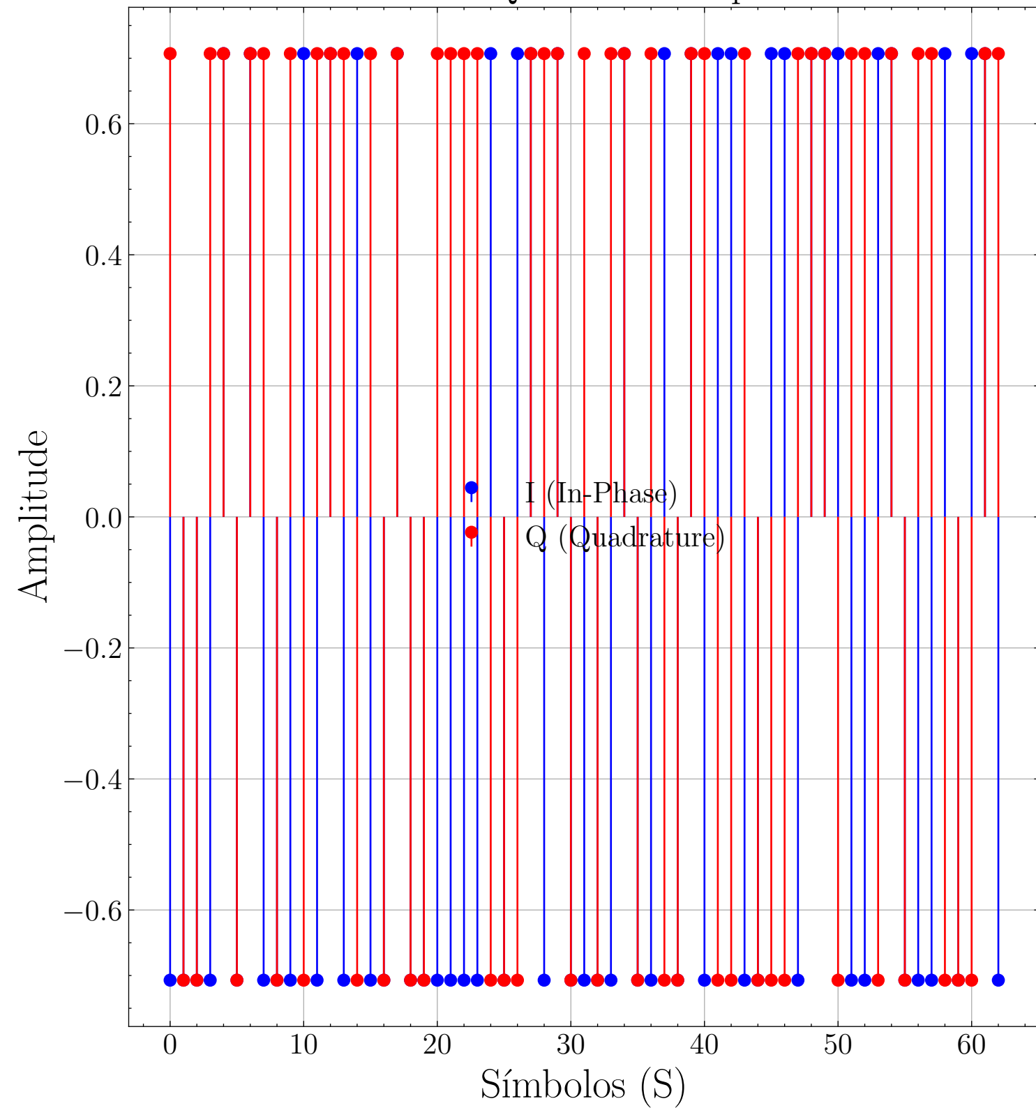
Sinal QPSK no Tempo
