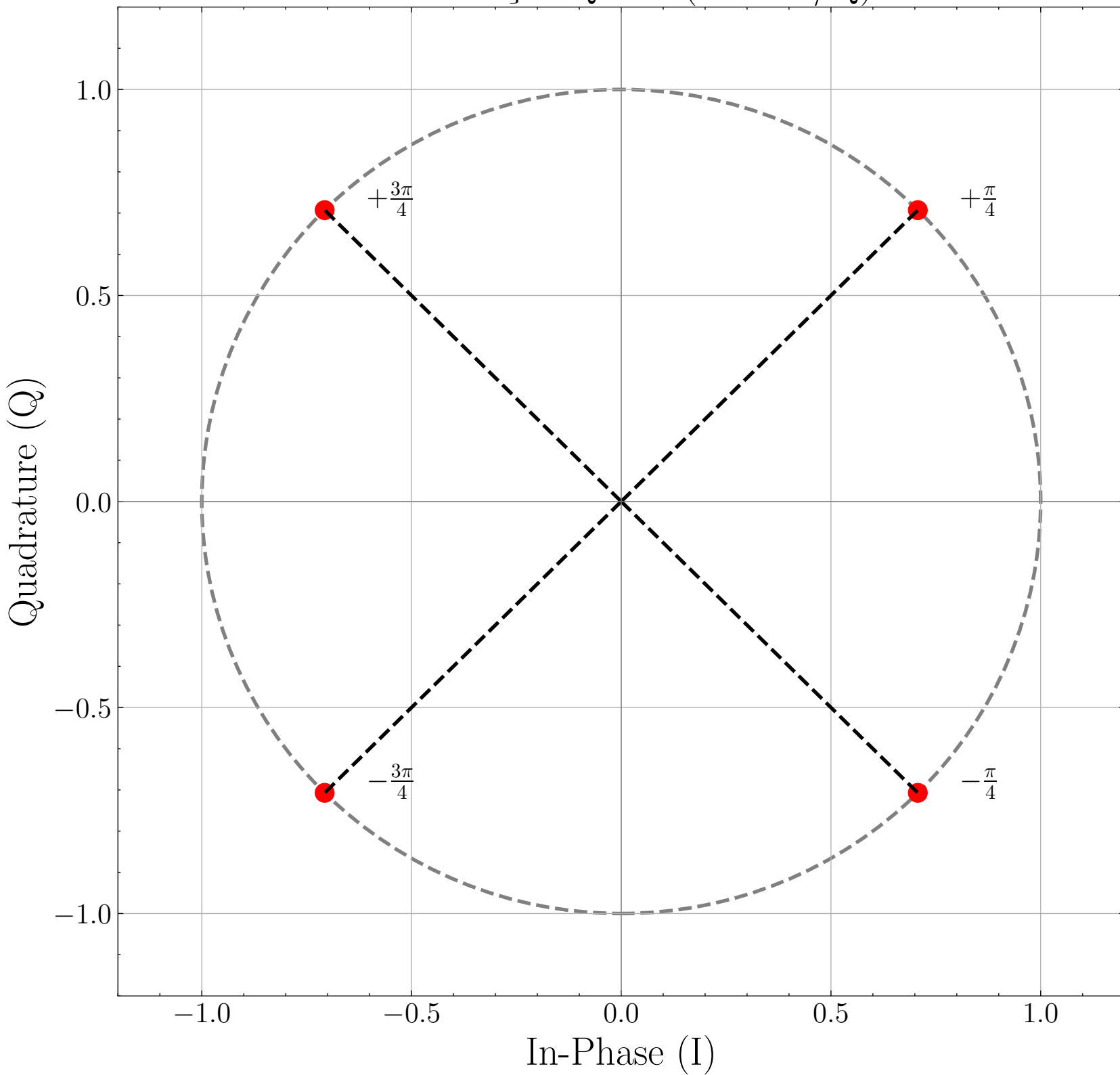
Constelação QPSK (Plano I/Q)
