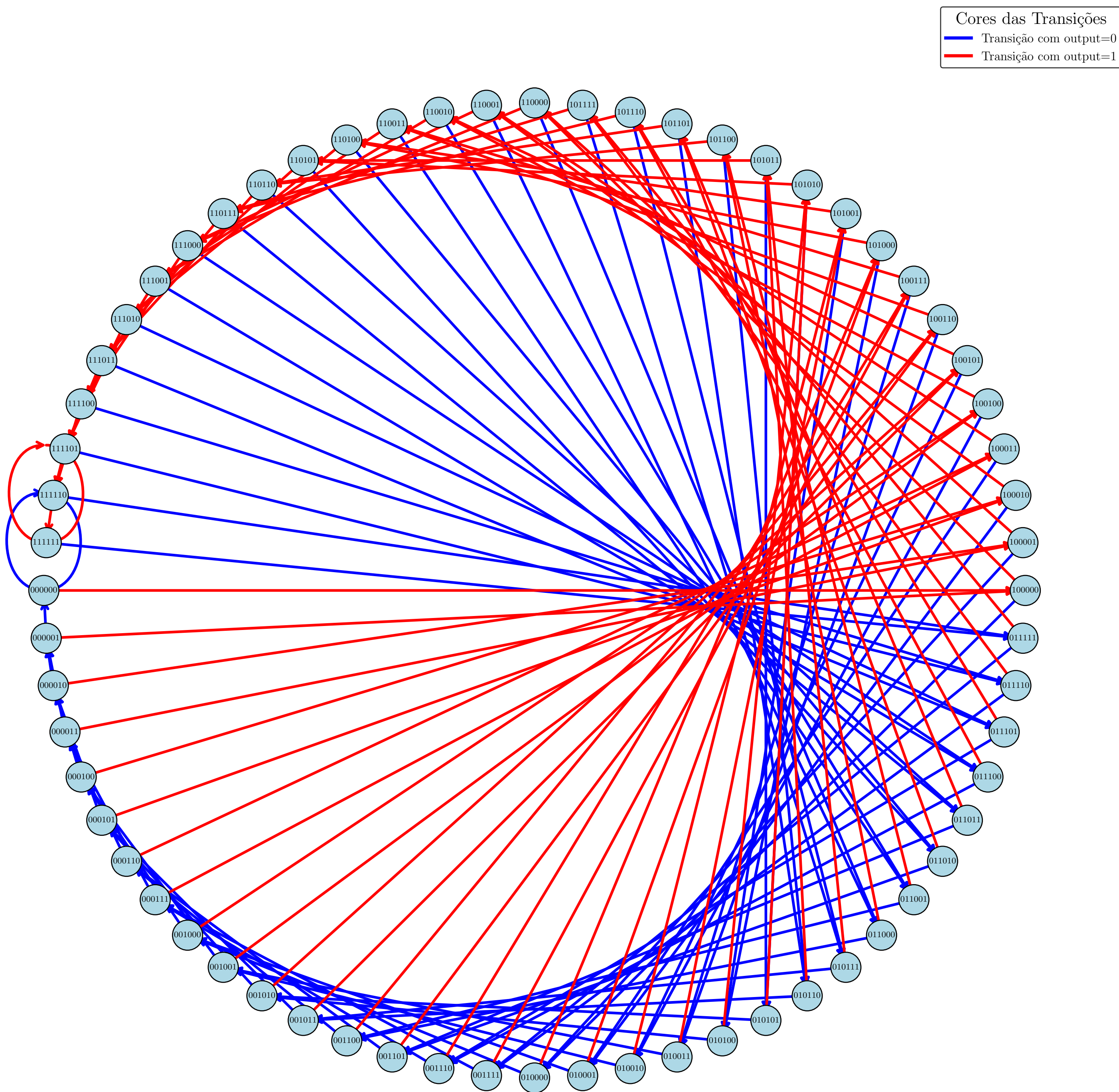
Trelha Completa do Codificador Convolucional (64 Estados, 128 Transições)
