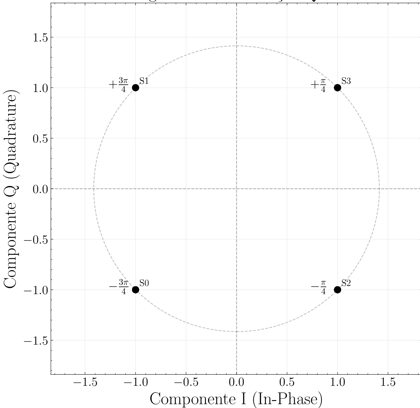
Diagrama de Constelação QPSK
