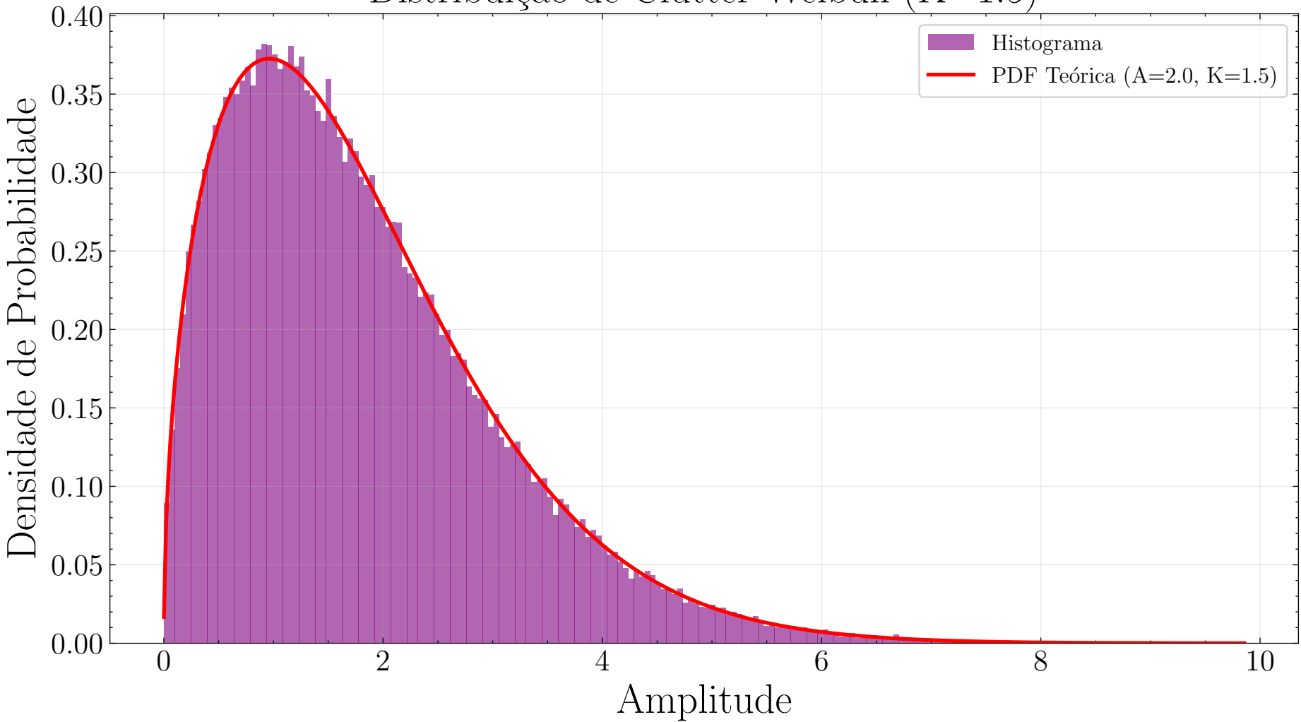
Distribuição de Clutter Weibull ( K=1.5 )
