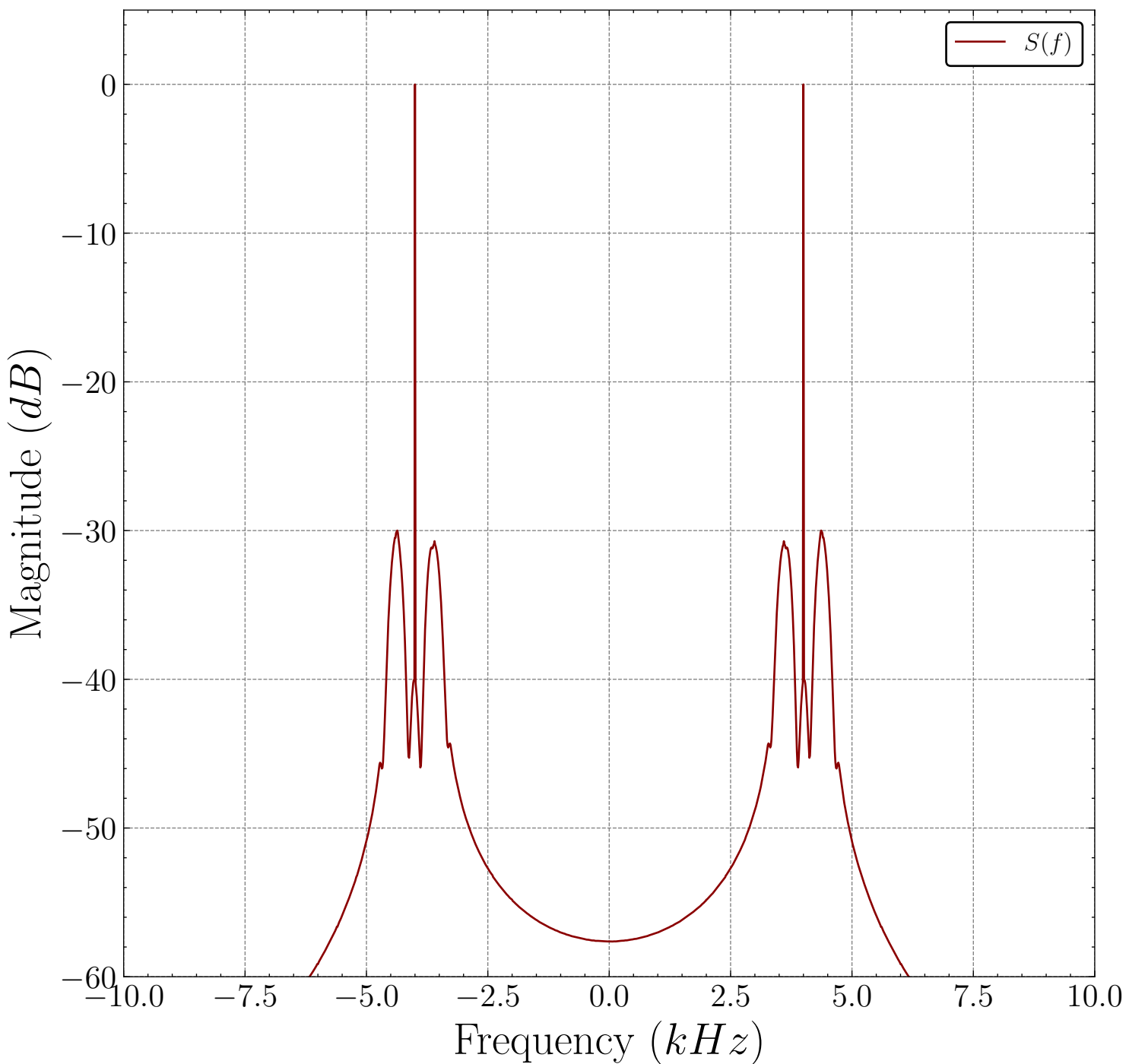
Portadora Pura - 0 a 80ms
