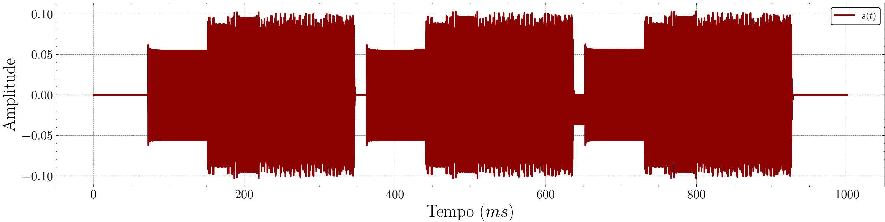
Sinal Modulado - Canal Total + Ruído
