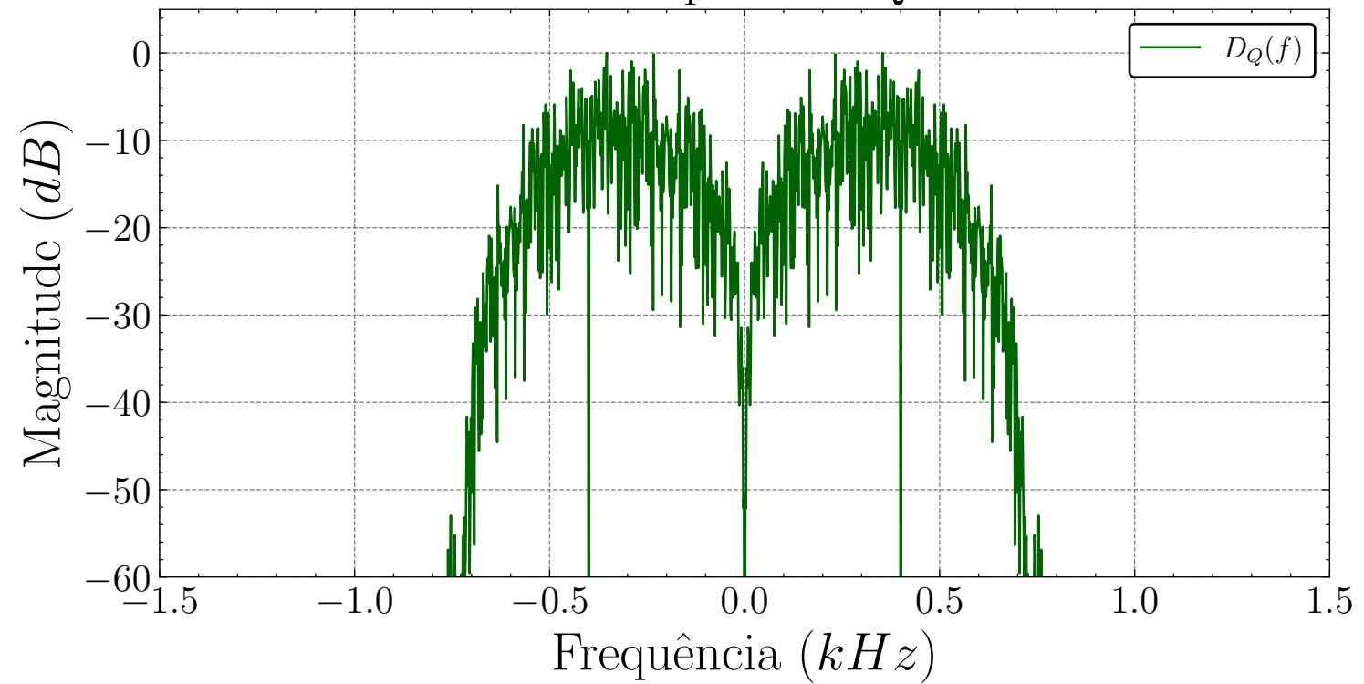
Sinal Modulado IQ
