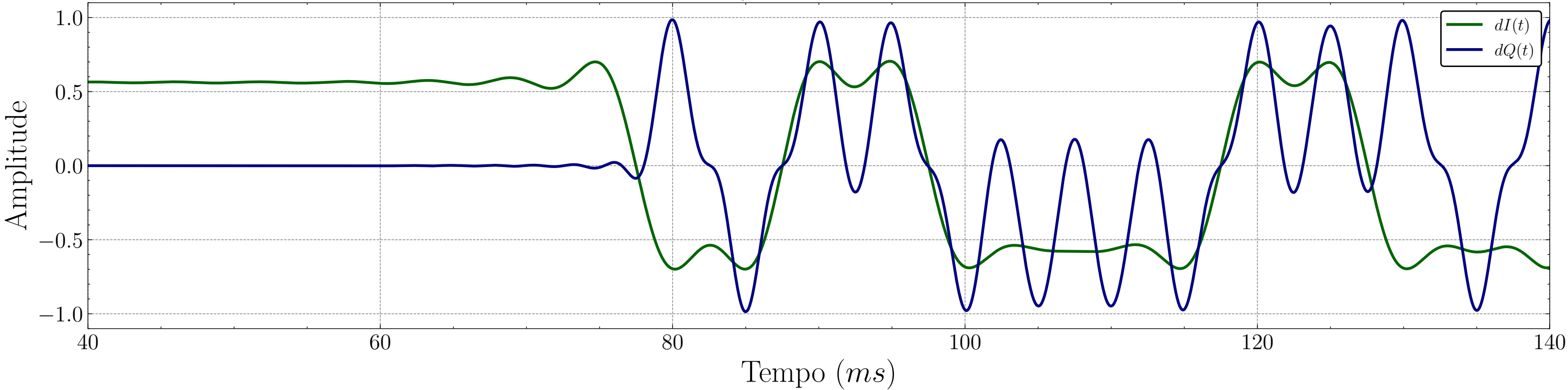
Sinal IQ - Formatados RRC
