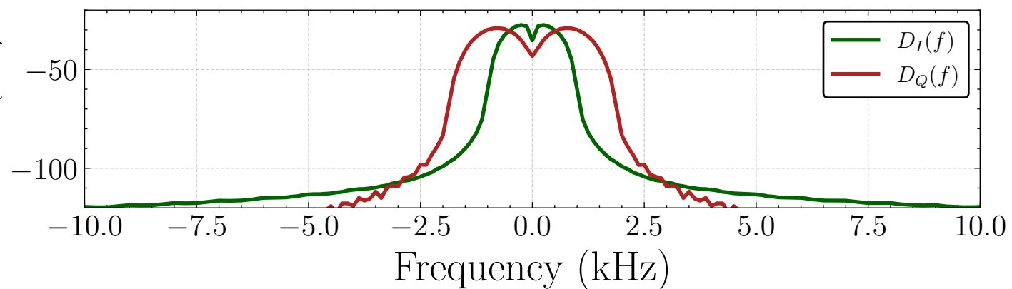
P. S. D. (dB/Hz)
