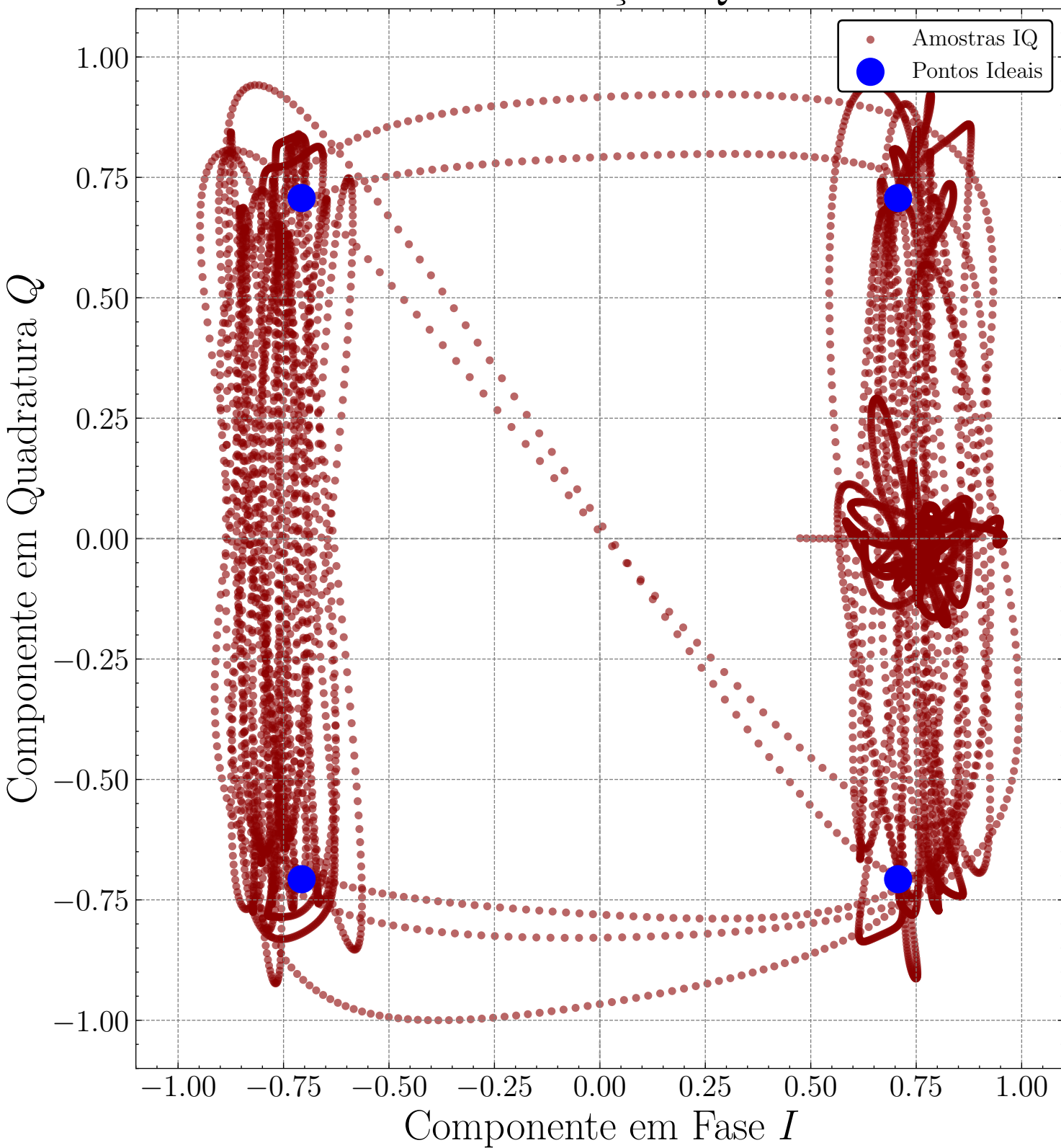
Constelação IQ
