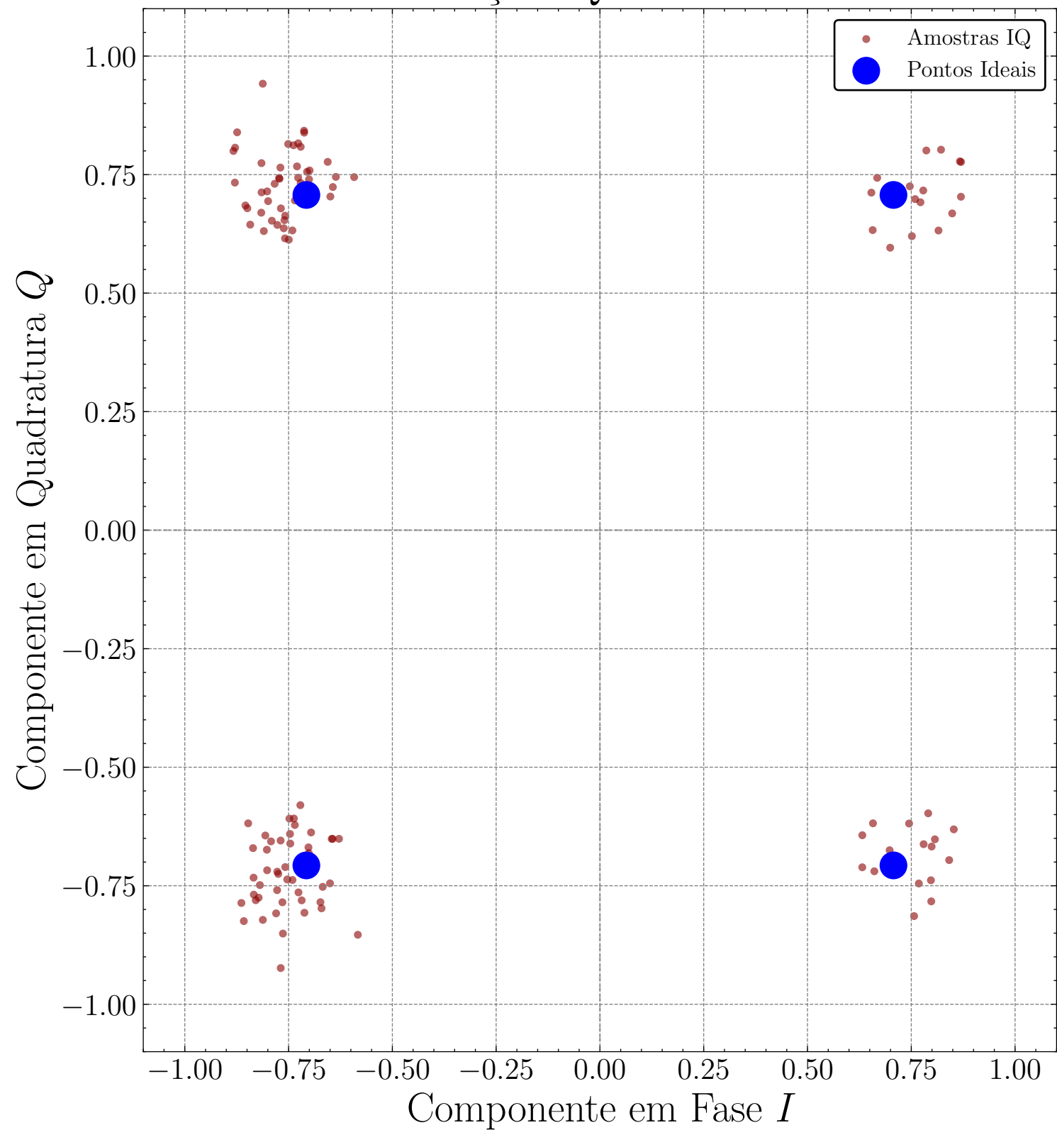
Constelação IQ – Amostrado
