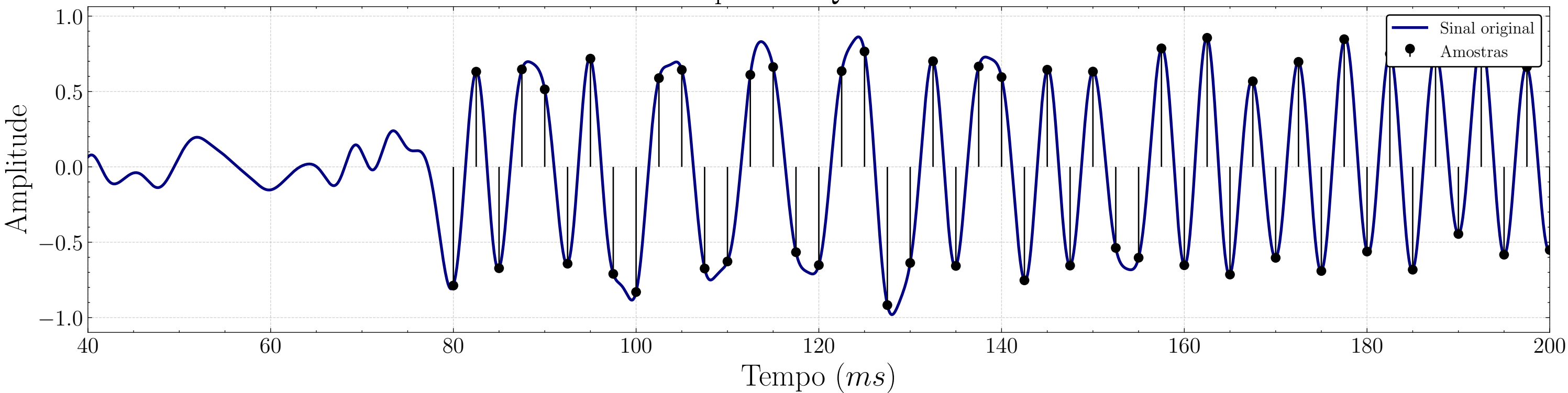
Componente Q amostrado
