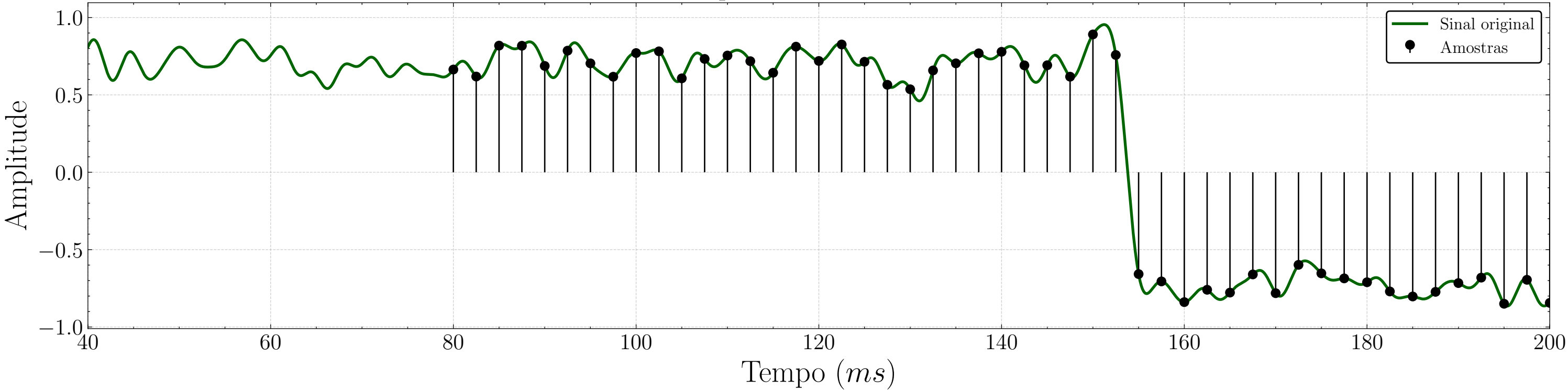
Componente I amostrado
