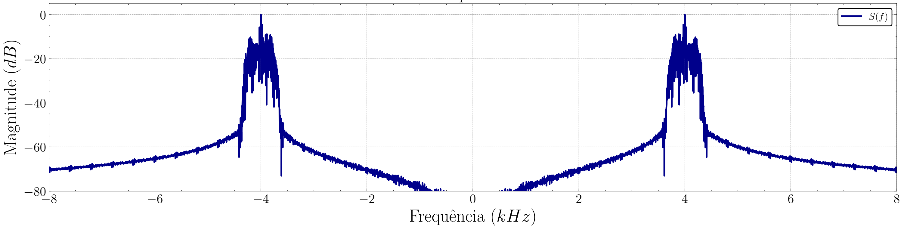
Domínio da Frequência - Com Ruído
