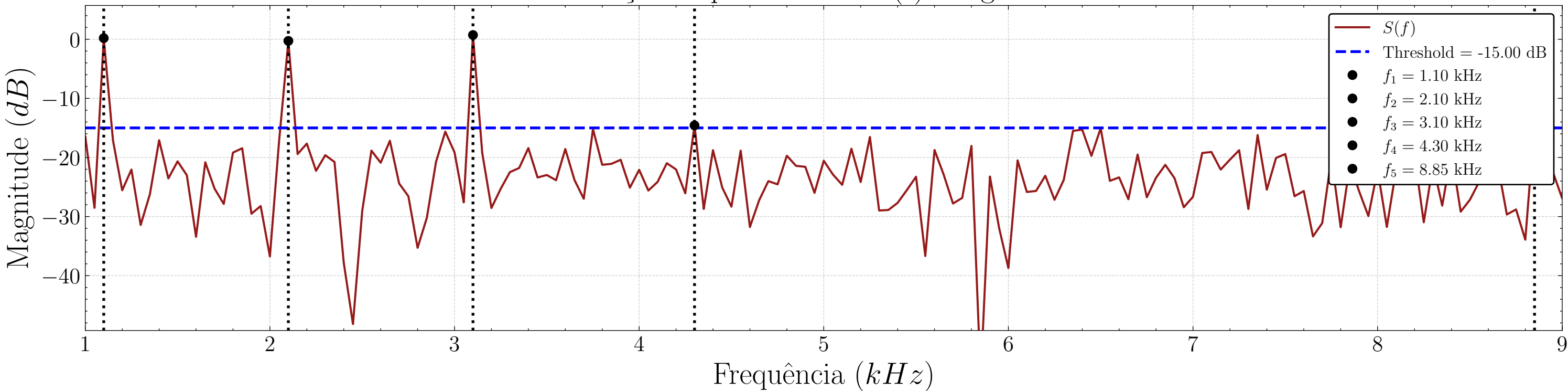
Detecção de portadora de s(t) - Segmento 1
