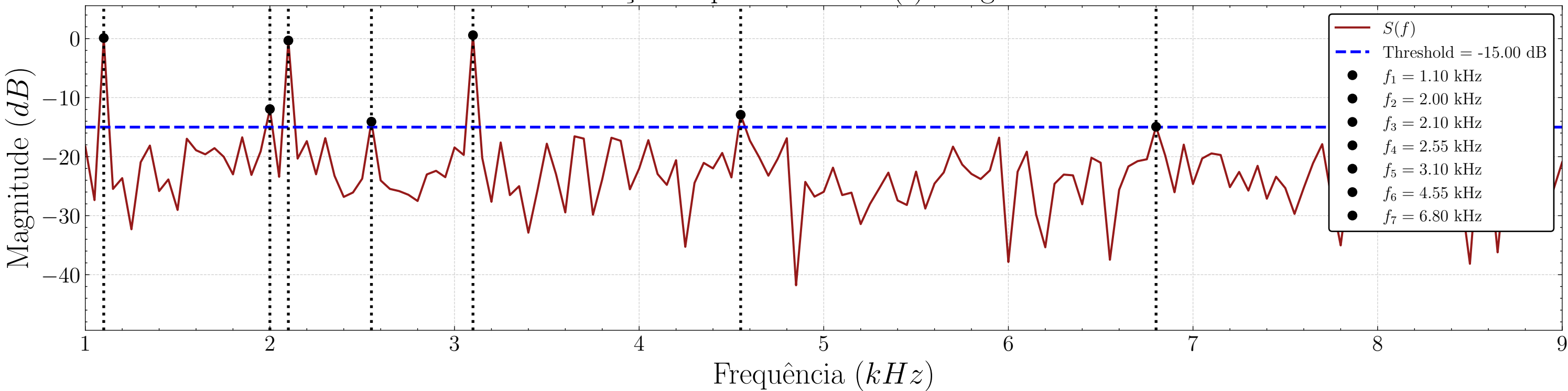
Detecção de portadora de s(t) - Segmento 2
