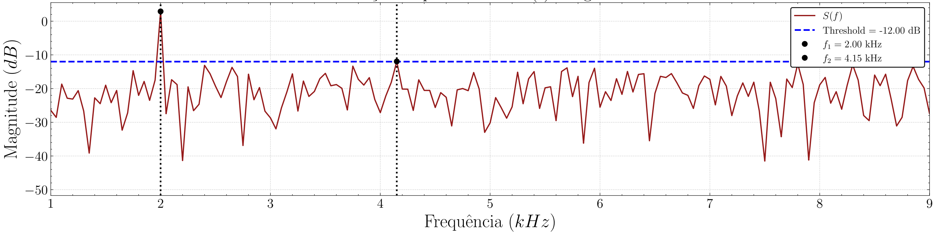
Detecção de portadora de s(t) - Segmento 5
