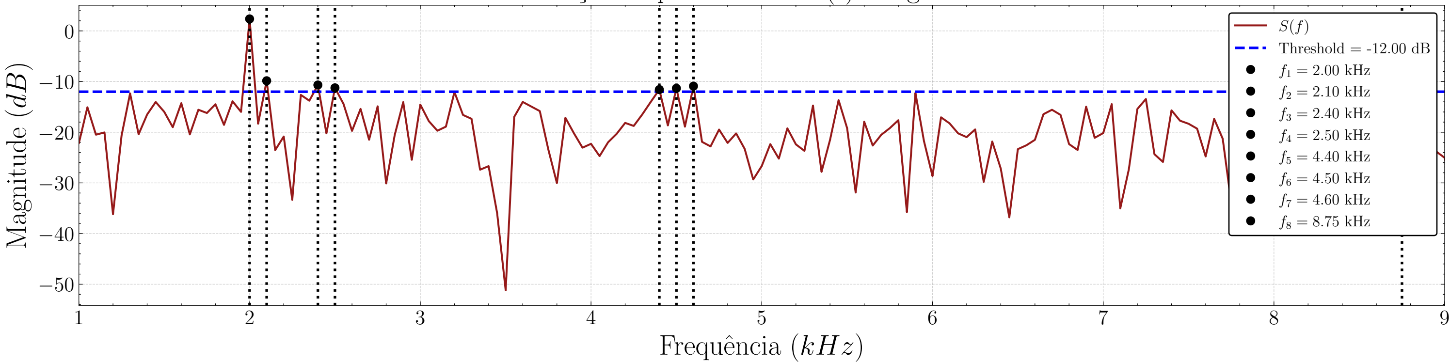
Detecção de portadora de s(t) - Segmento 6
