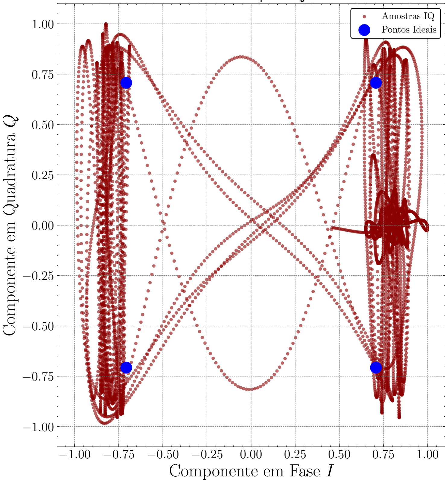
Constelação IQ
