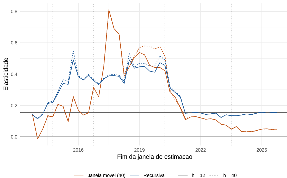
A. VAR estendido: elasticidade (resp. acum. fbcf_me / inf_diss)
