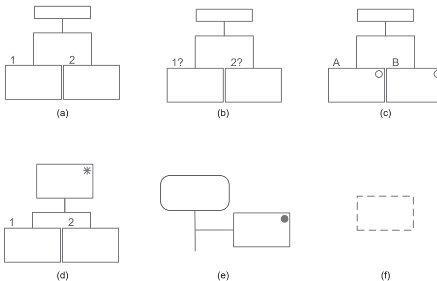
Figura 9.5: Representação de estrutura de tarefa: (a) sequencial, (b) independente de ordem, (c) alternativa, (d) iterativa, (e) ubíqua e (f) opcional.
