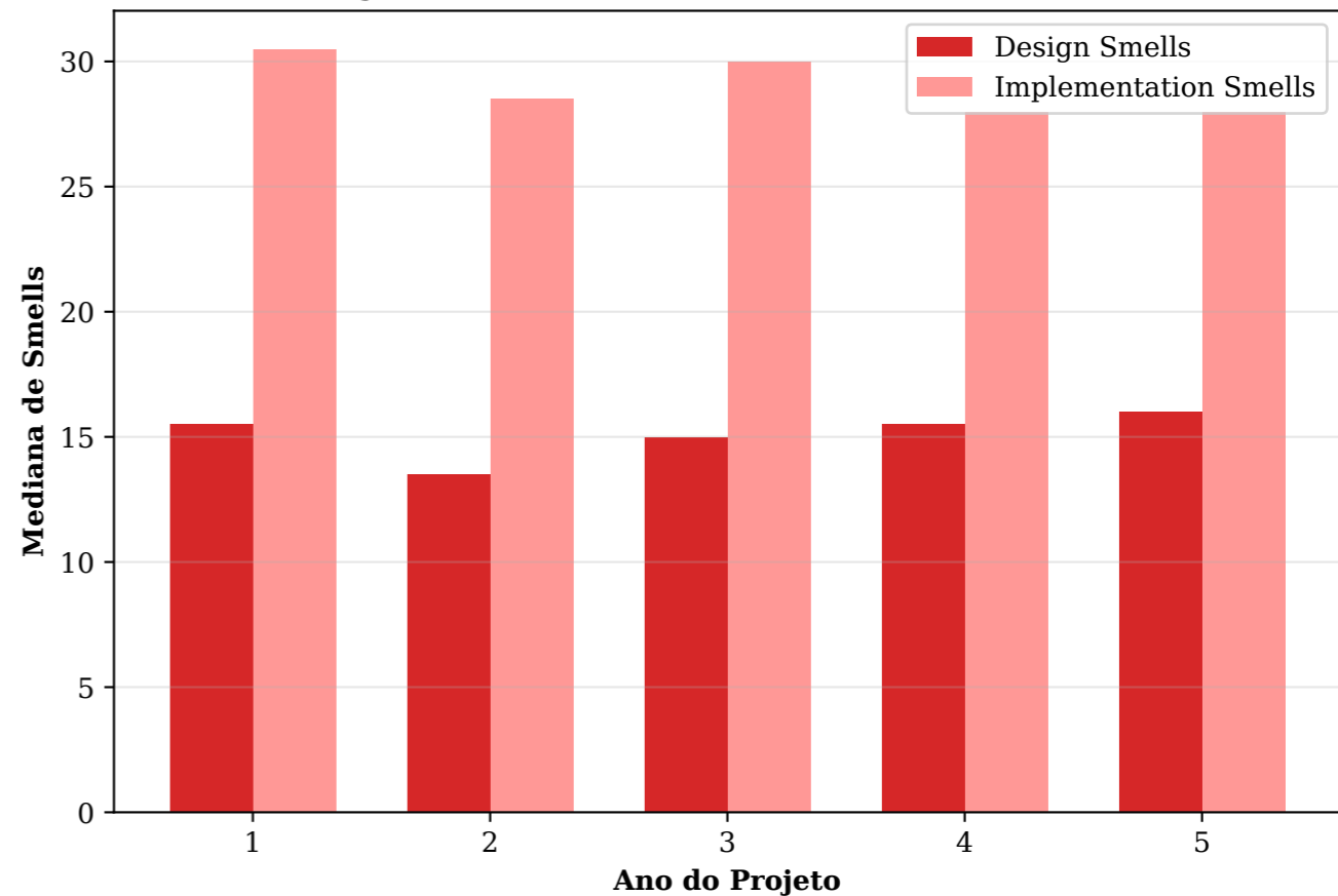
Design vs Implementation Smells - Mediana por Ano
