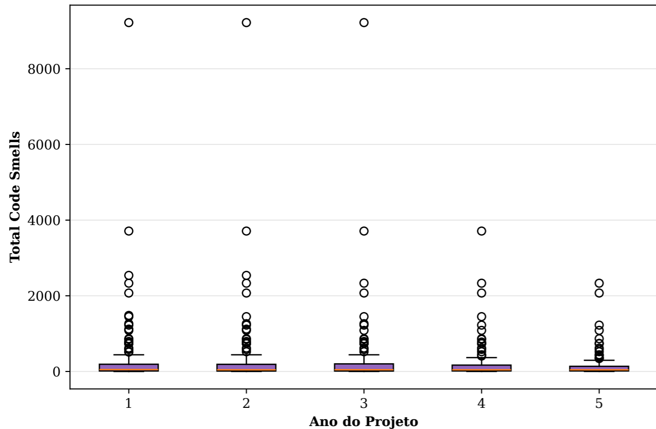
Distribuição Total de Code Smells por Ano
