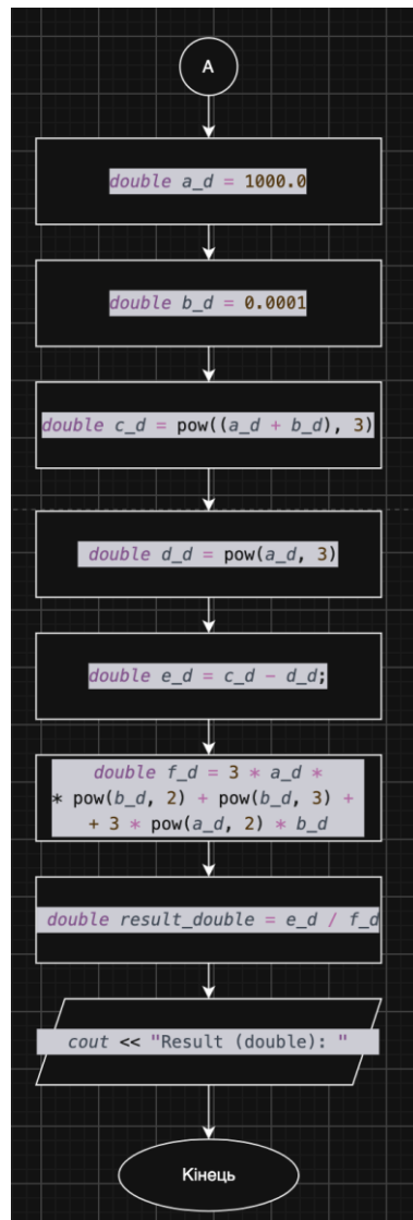
Рис 7. Блок-схема до задачі lab 1 task 1
