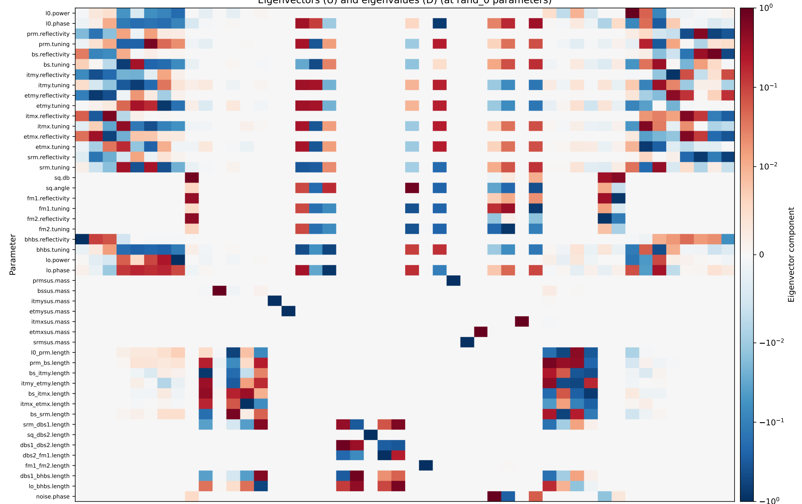
Eigenvectors (U) and eigenvalues (D) (at rand_0 parameters)
