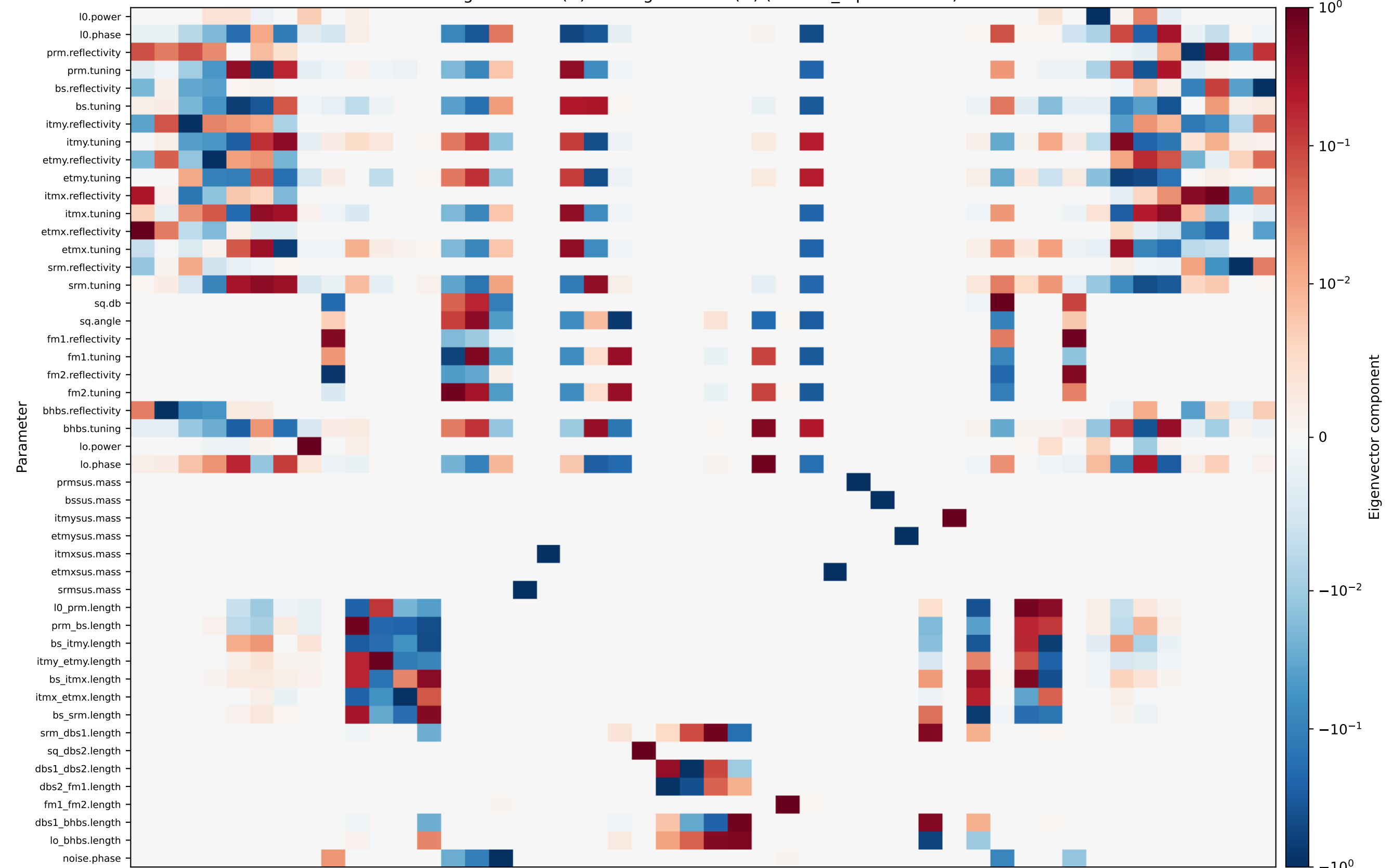
Eigenvectors (U) and eigenvalues (D) (at rand_2 parameters)
